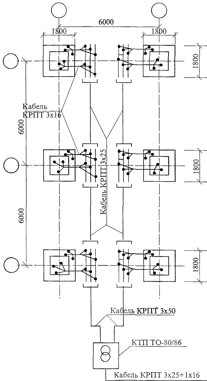
Рисунок 4 – Схема подключения шинпроводов к питающей сети
