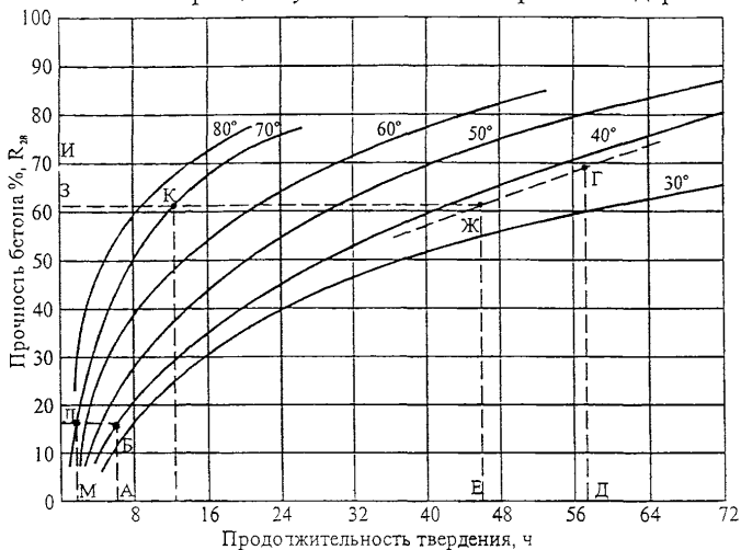
Рисунок 9 – Пример определения прочности бетона по графику
