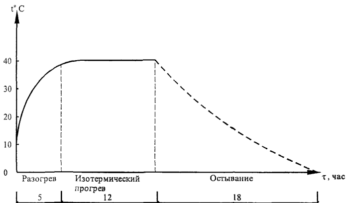
Рисунок 7 – График температурного режима электродного прогрева конструкции
