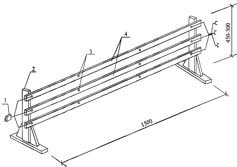
1 – разъем; 2 – деревянная стойка; 3 – болты; 4 – токопроводы (полоса 3×40 мм)
