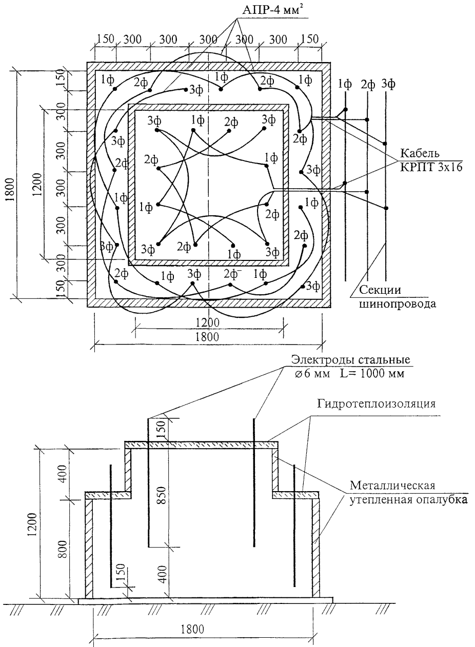
Рисунок 3 – Схема установки электродов и подключения к шинпроводам
