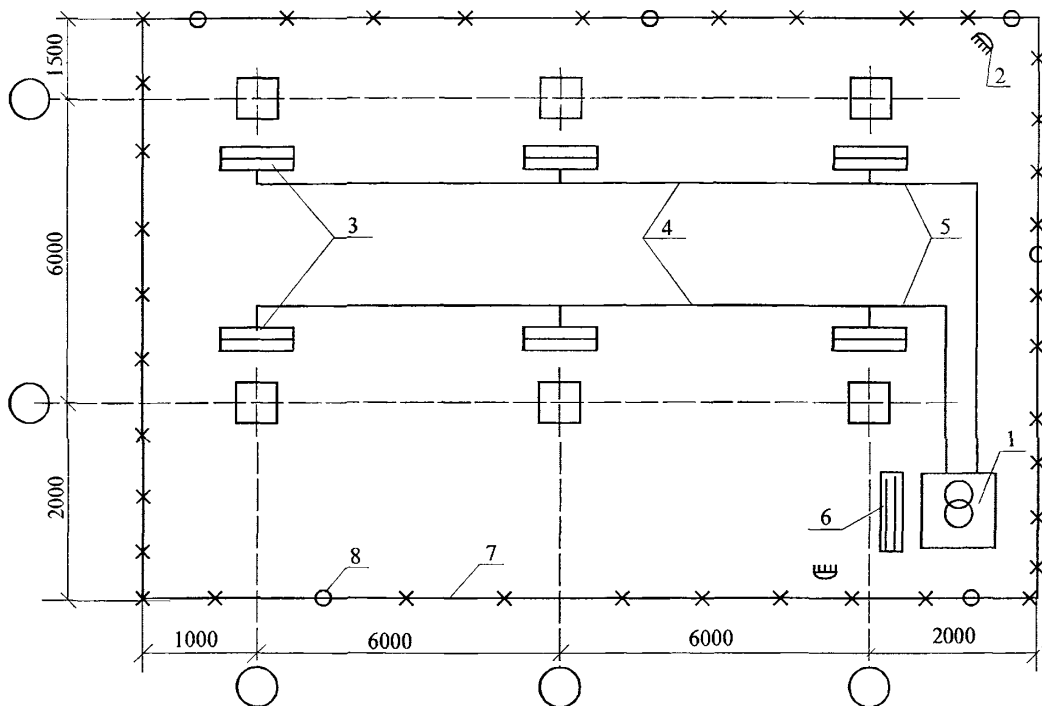
1 – комплектная трансформаторная подстанция КТП ТО-80/86; 2 – прожектор; 3 – секции шинопровода; 4 – кабель КРПТ 3×25; 5 – кабель КРПТ 3×50; 6 – диэлектрический коврик; 7 – инвентарные ограждения; 8 – сигнальная лампа красного цвета.
