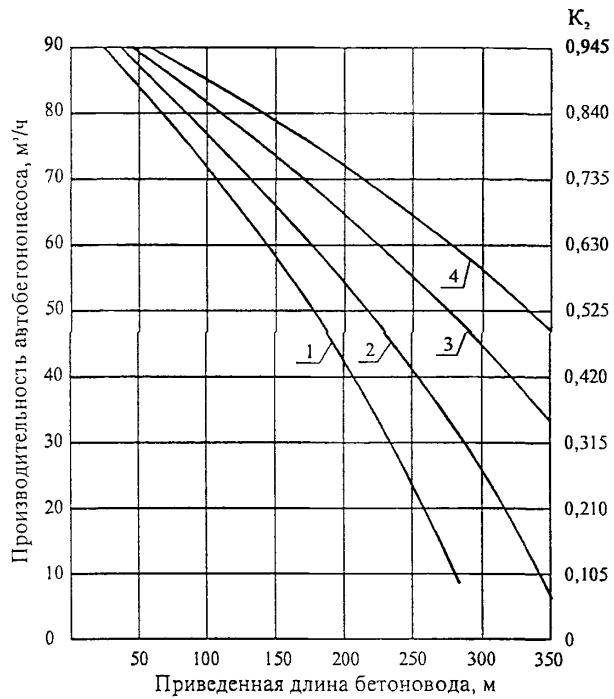
Рисунок 17 – Изменение производительности автобетононасоса фирмы «Томсен» модели 875 в зависимости от длины бетонорода
