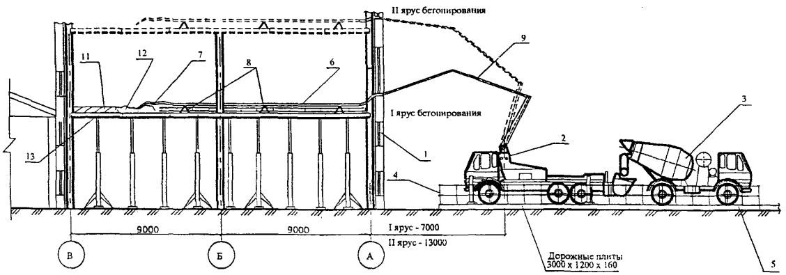
Рисунок 12 – Укладка бетонной смеси в перекрытие
