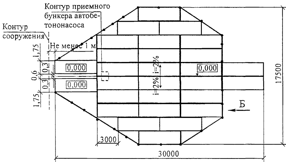
Рисунок 22 – Схема размещения комплекта машин при производстве бетонных работ на объекте
