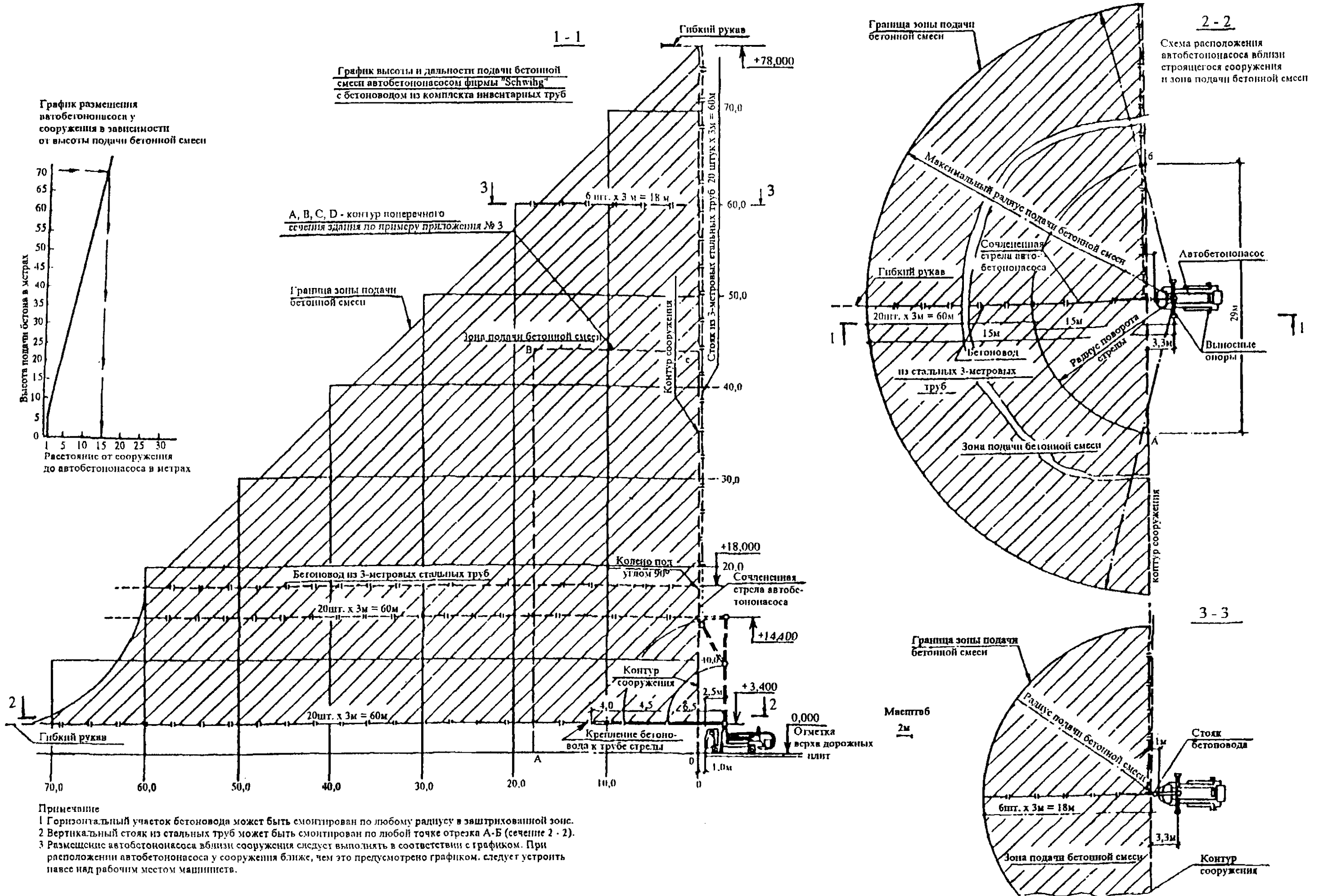
Рисунок 8 – Возможные зоны подачи и распределения бетонной смеси с одной стоянки автобетононасоса фирмы «SCHWING»
