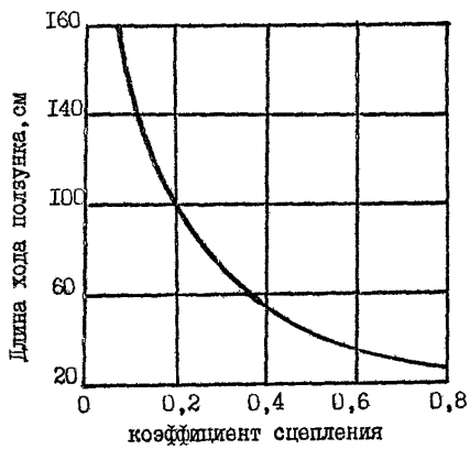
Рис.2. Зависимость между длиной хода ползунка прибора ППС-1 и коэффициентом сцепления на асфальтобетонном покрытии
