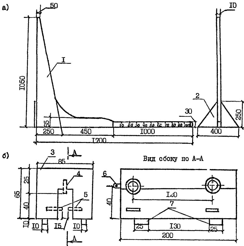
Рис. I. Портативный прибор для определения скользкости дорожных покрытий ПНС-I
