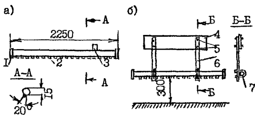
Рис. Распределительное устройство к поливочной машине для розлива жидких хлоридов:
