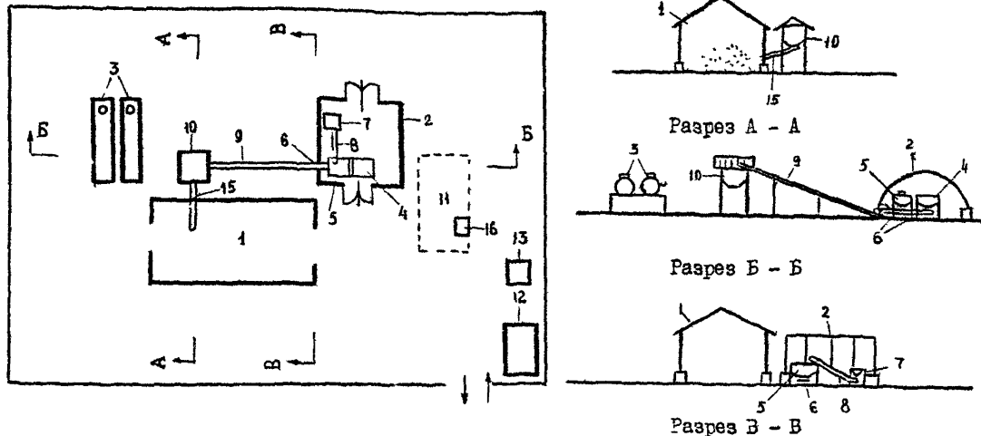
Рис. ПРИНЦИПИАЛЬНАЯ СХЕМА ЗАВЫ ПРОТИВОГОЛОЛЕДНЫХ МАТЕРИАЛОВ В РАВНИННОЙ МЕСТНОСТИ
