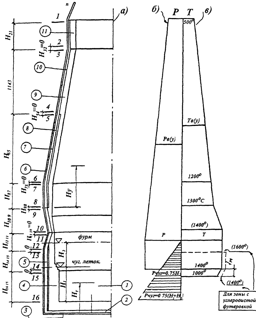
Рис. 7.1 Расчетная схема доменной печи
