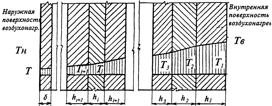
Рис. 7.5 Изменение температуры по толщине стенки воздухонагревателя
