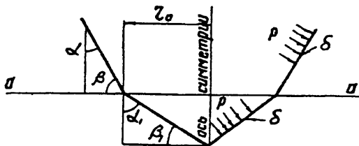
Рис. а Схема пересечения конусов
