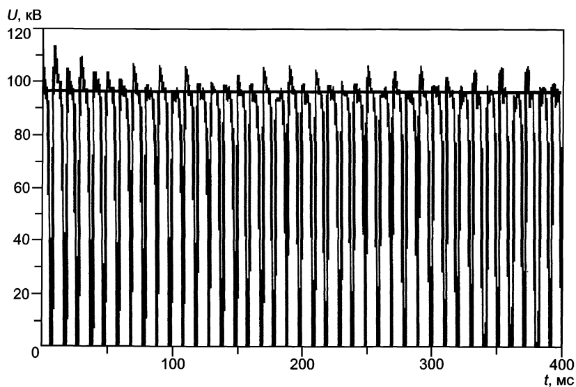
Рисунок В.1 — Пример выходного напряжения для двупульсного генератора
