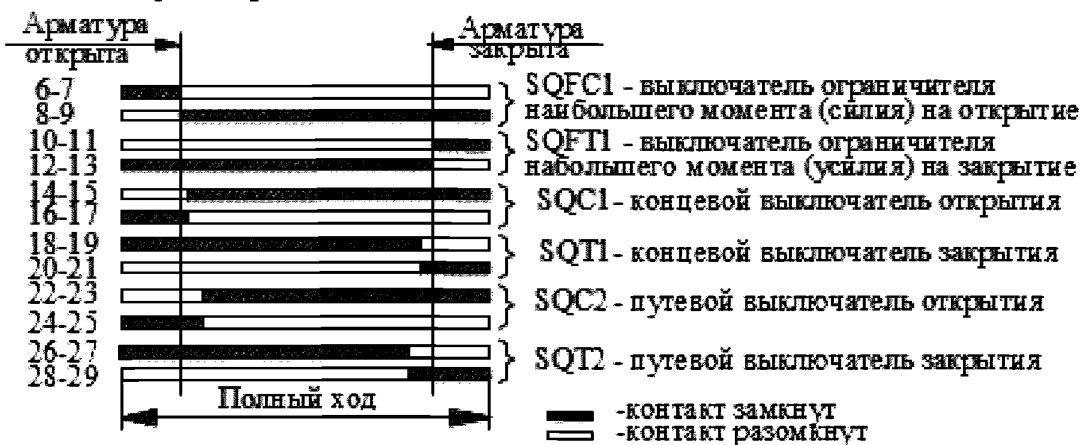
Диаграмма работы выключателей
