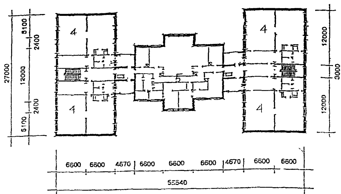
Рис 52 Детское дошкольное учреждение на 12 групп с плавательным бассейном (МНИИГЭП)
