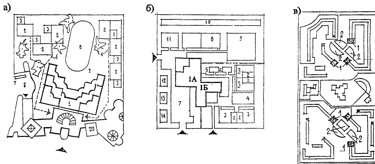
Рис. 2 Примеры решения участков в нестандартной ситуации
