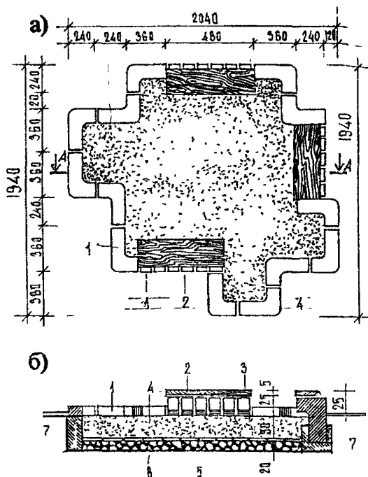
Рис. 11 Пример решения песочного дворика (опыт Болгарии) а - план; б - разрез
