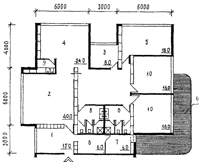
Рис. 37 Пример планировочного решения групповой ячейки детской группы с компенсирующей направленностью
