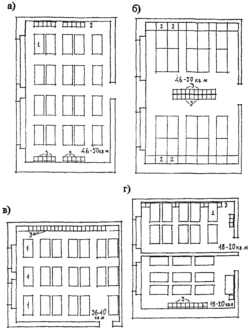
Рис. 34 Приемы размещения мебели в спальнях а - размещение в помещениях площадью 46-50 м 2 с индивидуальными кроватками; б - со встроенными откидными кроватками; в - размещение в одном помещении площадью 36-40 м 2 ; г - размещение с двумя подзонами по 18-20 м 2
