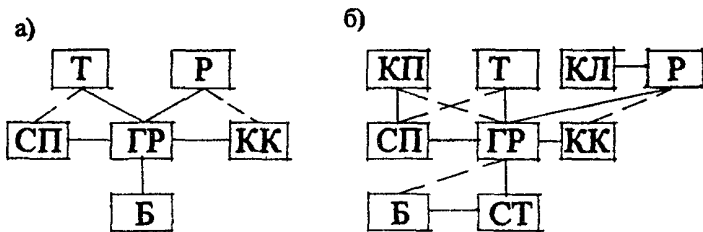
Рис. 36 Связи основных помещений компенсирующей групповой ячейки
