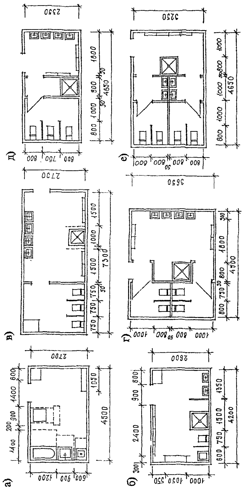
Рис. 35 Функционально-габаритные схемы туалетных а - детей 0-1 года; б - детей от 1 до 3 лет; в - детей от 3 до 5 лет; г, д, е - для детей 5-6(7) лет
