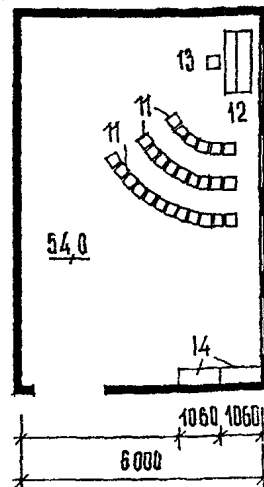
Рис. 40 Расстановка оборудования в залах для музыкальных и физических занятий а - для физических занятий площадью 100 м 2 ; б - то же, площадью 75 м 2 ; в - для музыкальных занятий 1 - стенка гимнастическая; 2 - канат; 3 - кольцо для пролезания; 4 - мостик-качалка; 5 - скамья гимнастическая; 6 - стойка для игровых пособий; 7 - стойка для прыжков; 8 - бревно гимнастическое; 9 - бревно круглое; 10 - шкаф для спортивного инвентаря; 11 - стул детский; 12 - пианино; 13 - табурет для пианино; 14 - шкаф для пособий
