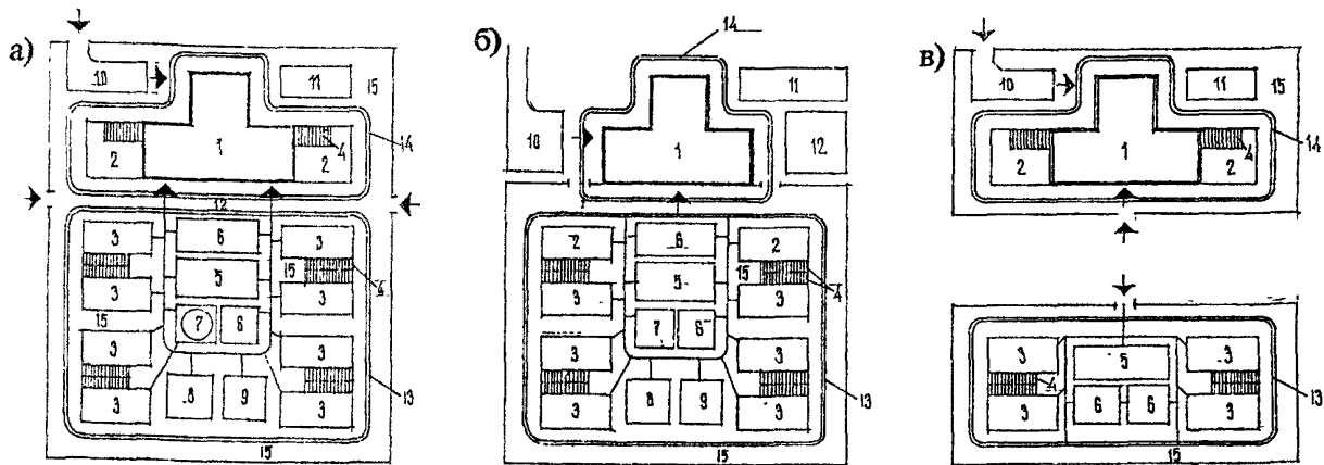
Рис. 1 Принципиальные схемы решения участков ДУ
