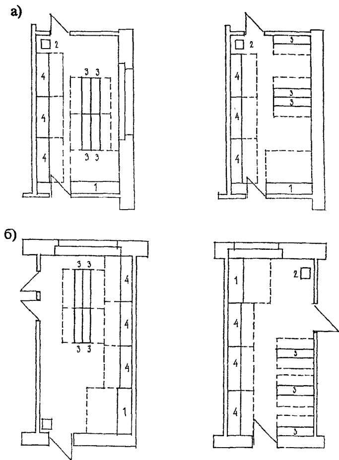
Рис. 27 Примеры размещения мебели в раздевальных: а - группы детей 2-3 лет; б - детей 3-6(7) лет 1 - шкаф для одежды персонала; 2 - табурет; 3 - скамья для переодевания, детская; 4 - шкаф для детской одежды
