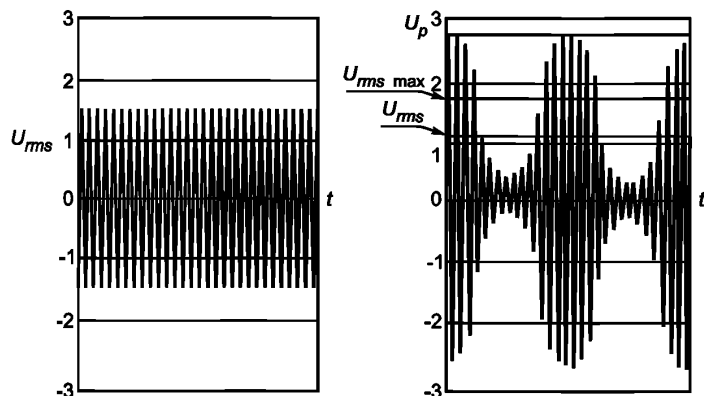
а) Немодулированный радиочастотный сигнал (пиковое значение напряжения U_p = 1,4 В, среднеквадратическое значение напряжения U_{rms} = 1 В);
