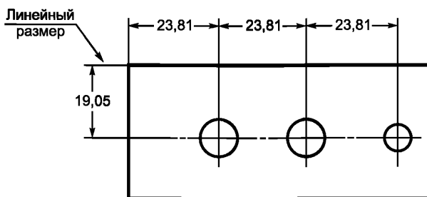
Рисунок 7 — Группа последовательных размеров
