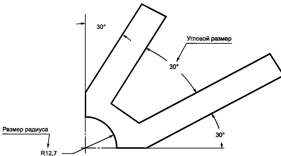
Рисунок 1 — Размеры угла и радиуса
