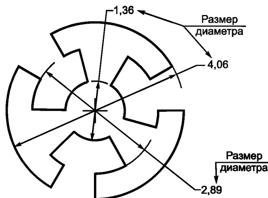
Рисунок 4 — Размер диаметра
