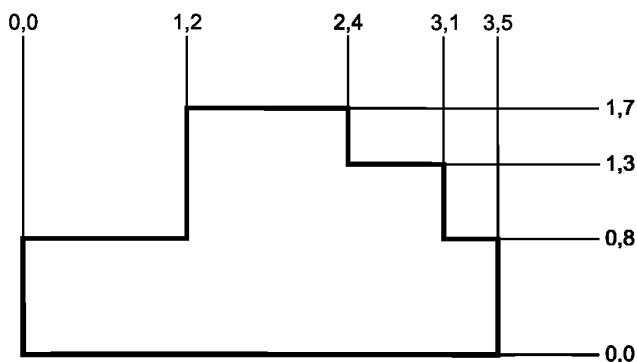
Рисунок 9 — Ординатный размер
