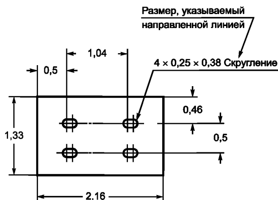
Рисунок 8 — Размер, указываемый направленной линией
