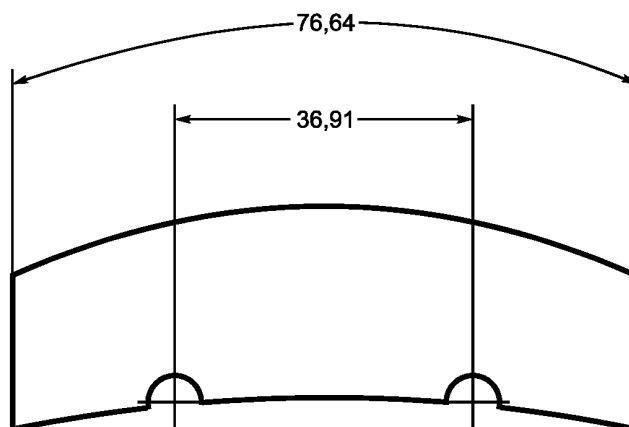
Рисунок 2 — Размер дуги
