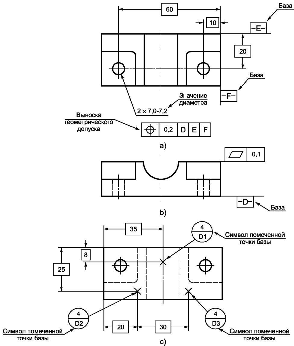
Рисунок 3 — Чертежные выноски
