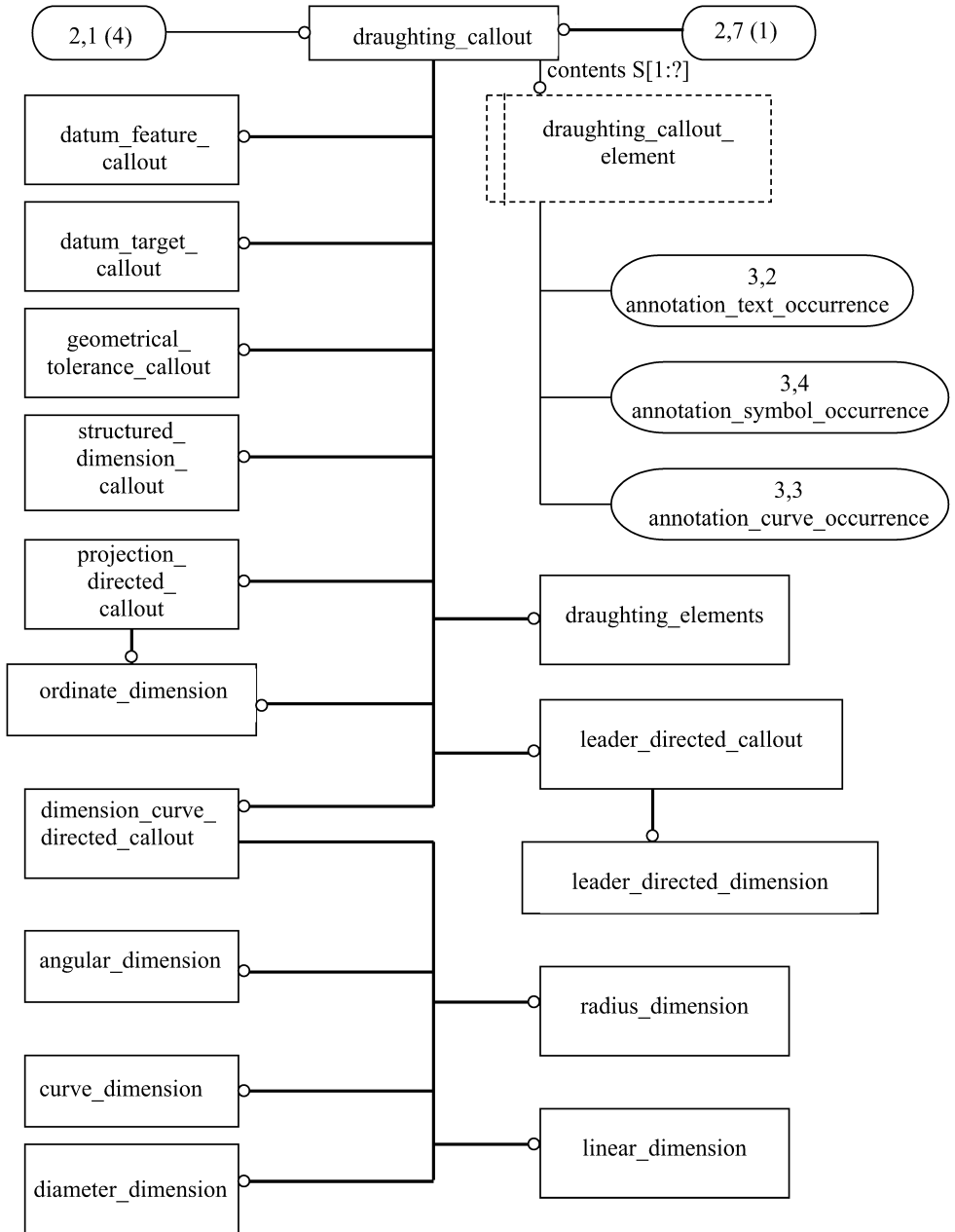
Рисунок С.2 — Расширенный листинг ПИК — EXPRESS-G-диаграмма 2 из 4
