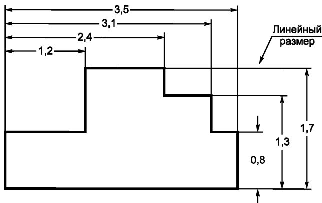
Рисунок 6 — Группы параллельных размеров
