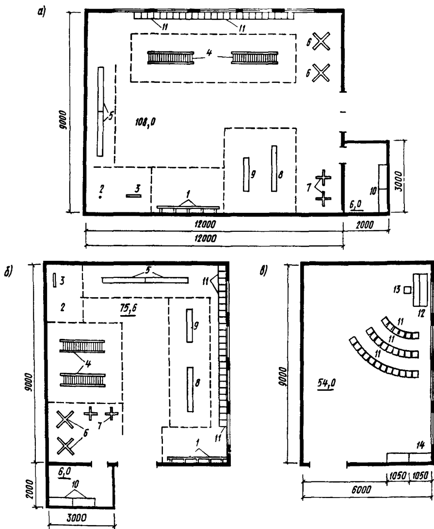
Рис. 44. Расстановка оборудования в залах
