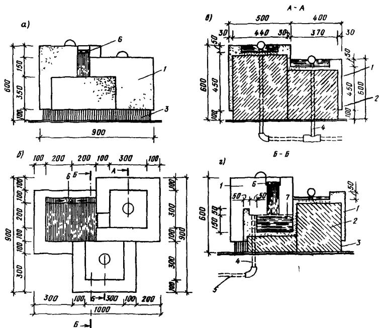
Рис. 24. Фонтанчики для игр с водой (опыт НРБ) а - фасад; б - план; в - разрез А-А; г - разрез Б-Б 1 - белая полированная мозаика; 2 - бетон; 3 - черная тертая мозаика; 4 - труба; 5 - отводная труба; 6 - водослив; 7 - латунная решетка
