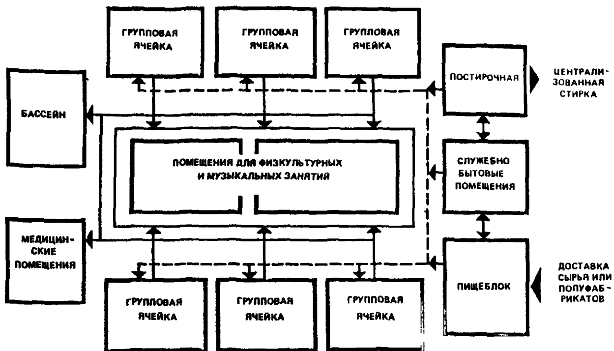
Рис. 31. Схема функциональной взаимосвязи групп помещений в дошкольном учреждении
