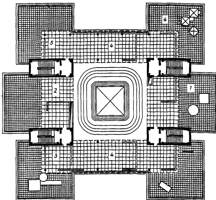
Рис. 17. Пример размещения групповых площадок на эксплуатируемой кровле здания. Комплекс яслей-сада на 480 мест в г. Ульяновске (ЦНИИЭП учебных зданий)
