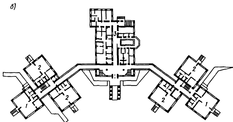
Рис. 1. Схема организации комплексов дошкольных учреждений (ЦНИИЭП учебных зданий) а - в виде отдельно стоящих зданий; б - в виде корпусов, соединенных переходом 1 - корпус ясельных групп; 2 - корпус групп детского сада; 3 - служебно-бытовое здание
