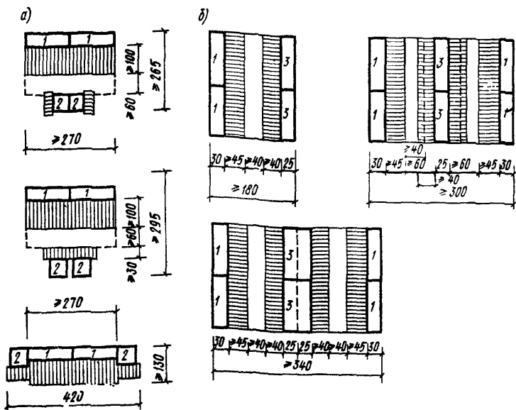
Рис. 35. Размещение оборудования с функциональными зонами в раздевальнях
