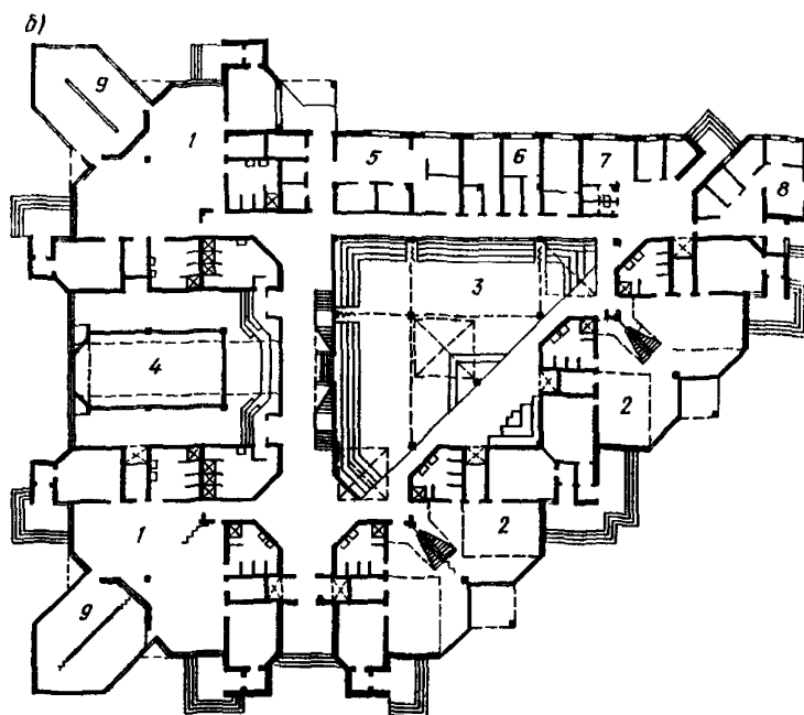
Рис. 8. Ясли-сад на 140 мест с сезонным расширением конкурсный проект, архитекторы С.Новоселов, Е.Смирнова) а - фасад; б - план первого этажа; в - план мансарды; 1 - помещения групп ясельного возраста; 2 - помещения групп дошкольного возраста; 3 - зал для гимнастических и музыкальных занятий; 4 - бассейн; 5 - кухня; 6 - постирочная; 7 - помещения администрации; 8 - медицинские помещения; 9 - летние стальные веранды ясельных групп; 10 - летние спальные веранды дошкольных групп
