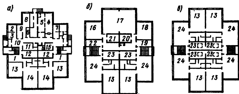
Рис. 32. Трехэтажное здание яслей-сада на 190 мест в конструкциях I.090.I-I в г.Калинине (ЦНИИЭП учебных зданий)
