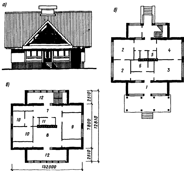
Рис. 6. Детский сад, совмещенный с квартирой для обслуживающего персонала, размещенной в мансарде (МосгипроНИИсельстрой) а - фасад; б - план первого этажа; в - план мансарды; помещения детского сада: 1 - приемная; 2 - спальня; 3 - игральня-столовая; 4 - кухня; 5 - постирочная; 6 - туалетная; помещения жилого дома: 7 - прихожая; 8 - кухня; 9 - общая комната; 10 - спальня; 11 - санузел; 12 - веранда
