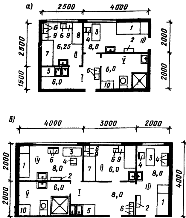
Рис. 48. Примеры планировки медицинских помещений в яслях-садах вместимостью
