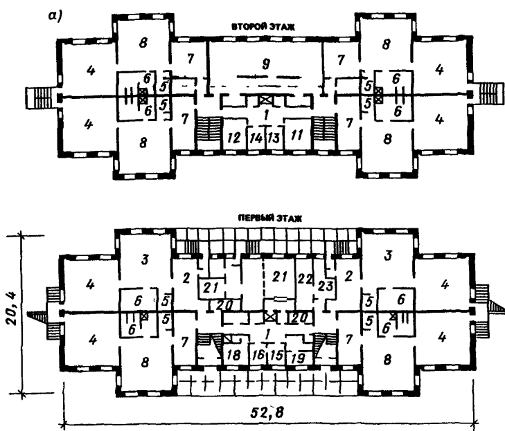
Рис. 28. Серия зданий яслей-садов в крупнопанельных конструкциях 1.090.1-1 (ЦНИИЭП учебных зданий)
