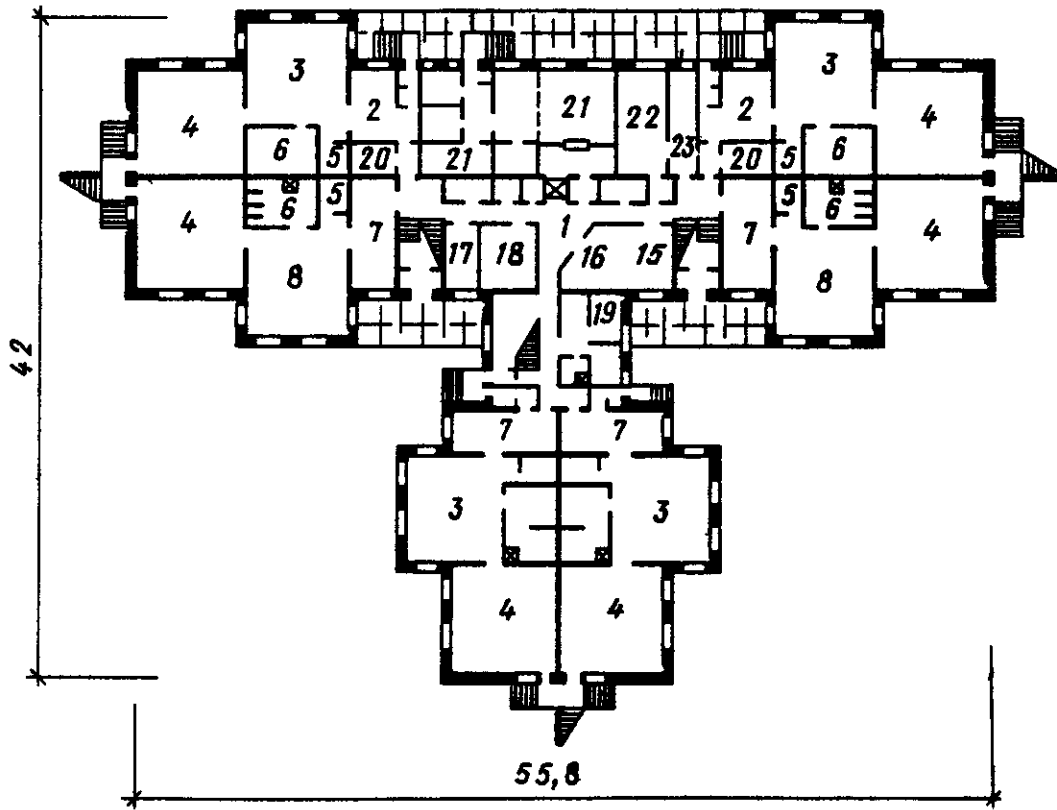
ПЕРВЫЙ ЭТАЖ
