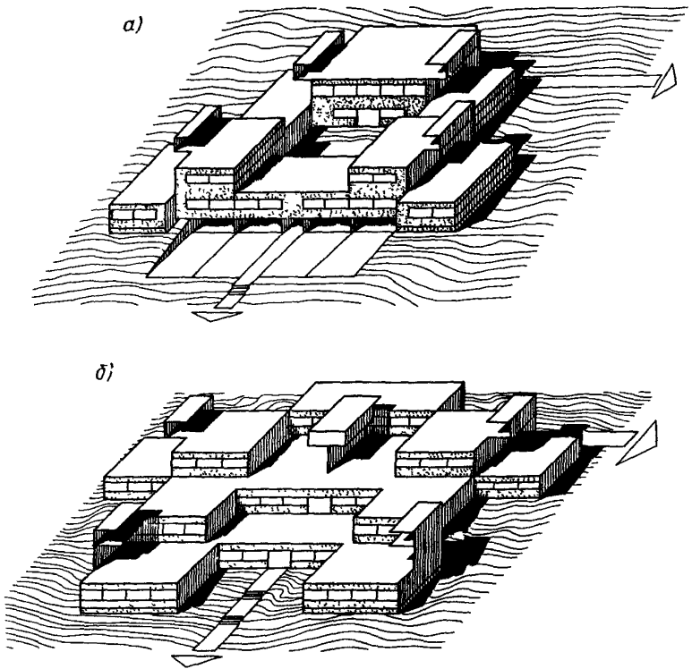
Рис. 10. Варианты решения зданий яслей-садов для размещения на рельефе (ЦНИИЭП градостроительства) а - с перепадом объемов в полэтажа на уклонах 10-35 %; б - террасного типа на уклонах 35-60 %
