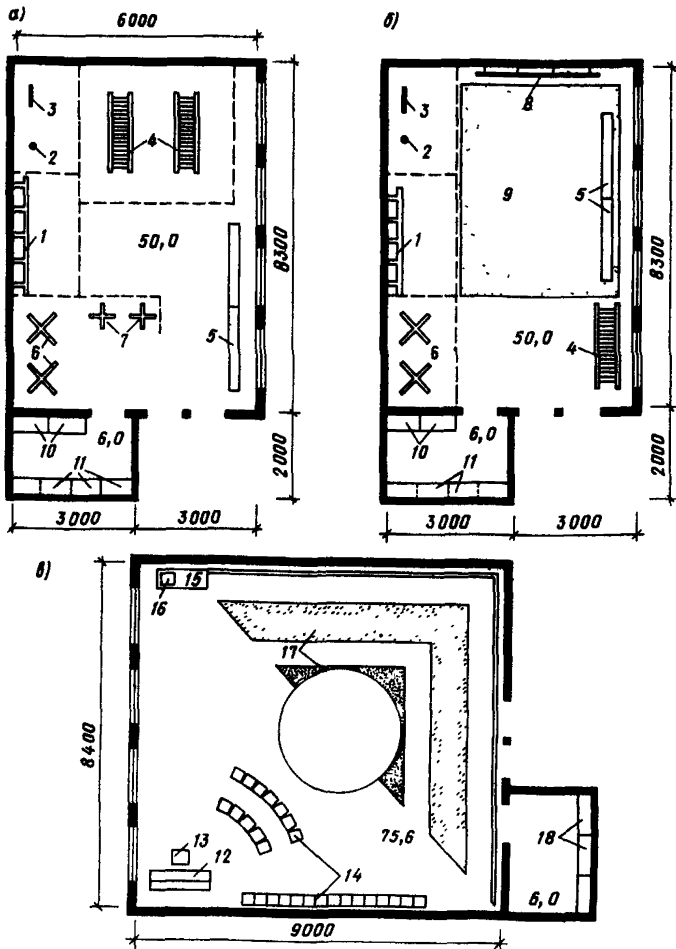
Рис. 45. Расстановка оборудования в залах специализированных детских учреждений
