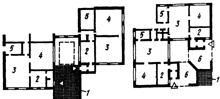
Рис. 37. Примеры организации мест для хранения колясок, санок, лыж
