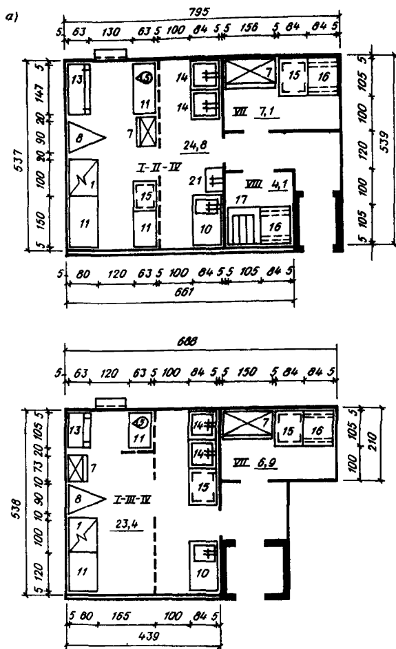
Рис. 49. Примеры планировок пищеблоков вместимостью а - до 50 мест; б - свыше 150 и до 250 мест; в - свыше 250 и до 350 мест; I - кухня с раздаточной; II - заготовочный цех; III - доготовочный цех; IV - моечная кухонной посуды; V - контейнерная; VI - охлаждаемые камеры с фреоновой установкой для хранения мясных и рыбных полуфабрикатов, овощных полуфабрикатов, молочных продуктов, жиров, гастрономии, мяса, рыбы; VII - кладовая сухих продуктов; VIII - кладовая овощей; IX - загрузоч-
