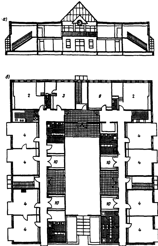
Рис. 26. Компактная схема объемно-планировочного решения здания детского сада на 170 мест (ДРГ)
