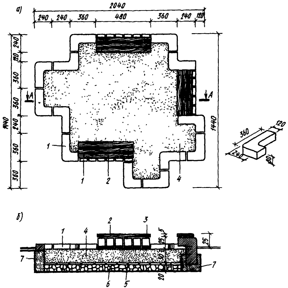
Рис. 20. Песочный дворик (опыт НРБ)
