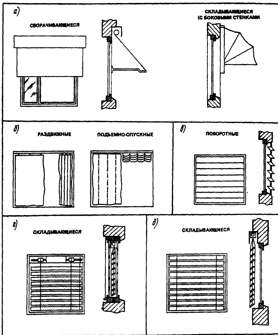
Рис. 33. Схемы СЗУ
