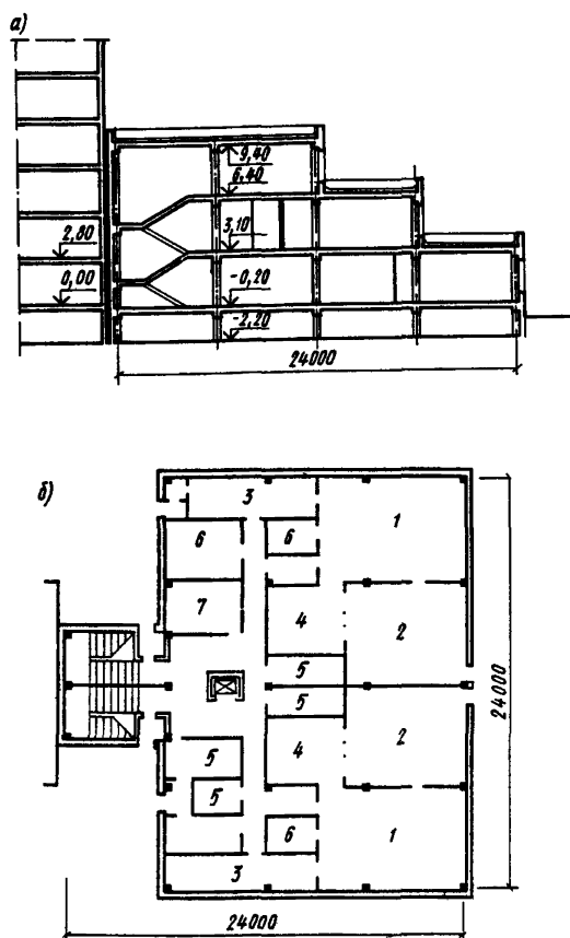
Рис. 30. Пример пристройки к жилому дому группового отделения детского сада на четыре группы в экспериментальном проекте комплекса дошкольного воспитания для микрорайона с высокой плотностью застройки и централизованным административно-хозяйственным обслуживанием (ЦНИИЭП учебных зданий)
