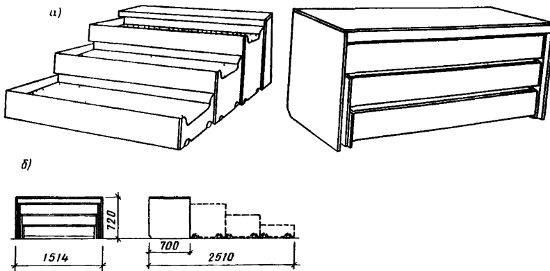
Рис. 41. Тумба-кровать трехъярусная (г. Минск)
