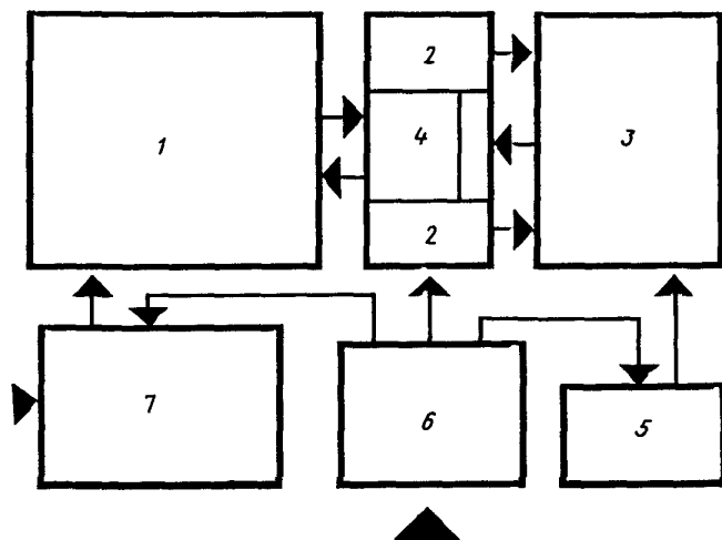
Рис. 46. Схема функциональной взаимосвязи помещений бассейна 1 - бассейн; 2 - раздевальня; 3 - зал для подготовительных занятий; 4 - душ; 5 - методический кабинет, класс; 6 - вес-тибюль; 7 - административно-бытовые помещения
