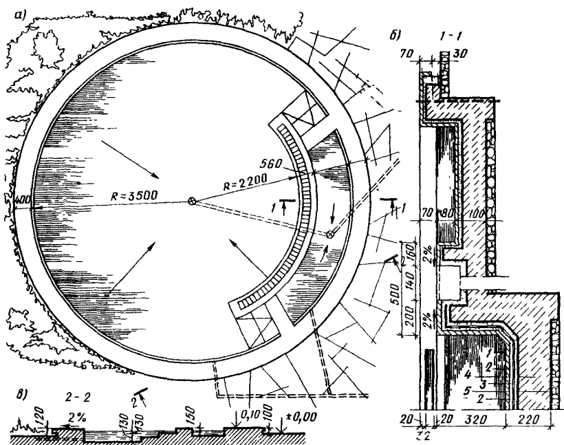
Рис. 23. Планировка и конструктивное решение песчаного бассейна (опыт НРБ) а - план; б - разрез 1-1; в - разрез 2-2; 1 - облицовочная плитка; 2 - цементная стяжка; 3 - гидроизоляция; 4 - бетон; 5 - дренаж
