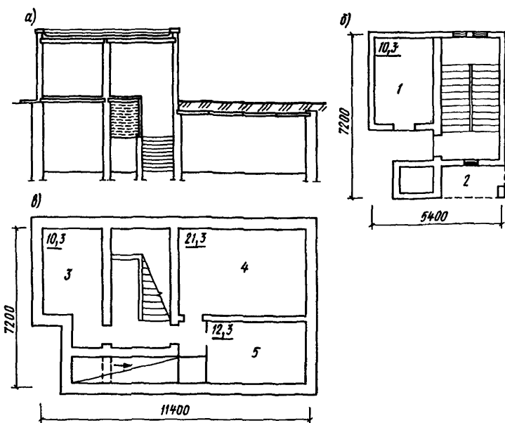
Рис. 25. Пример решения погреба-овощехранилища
