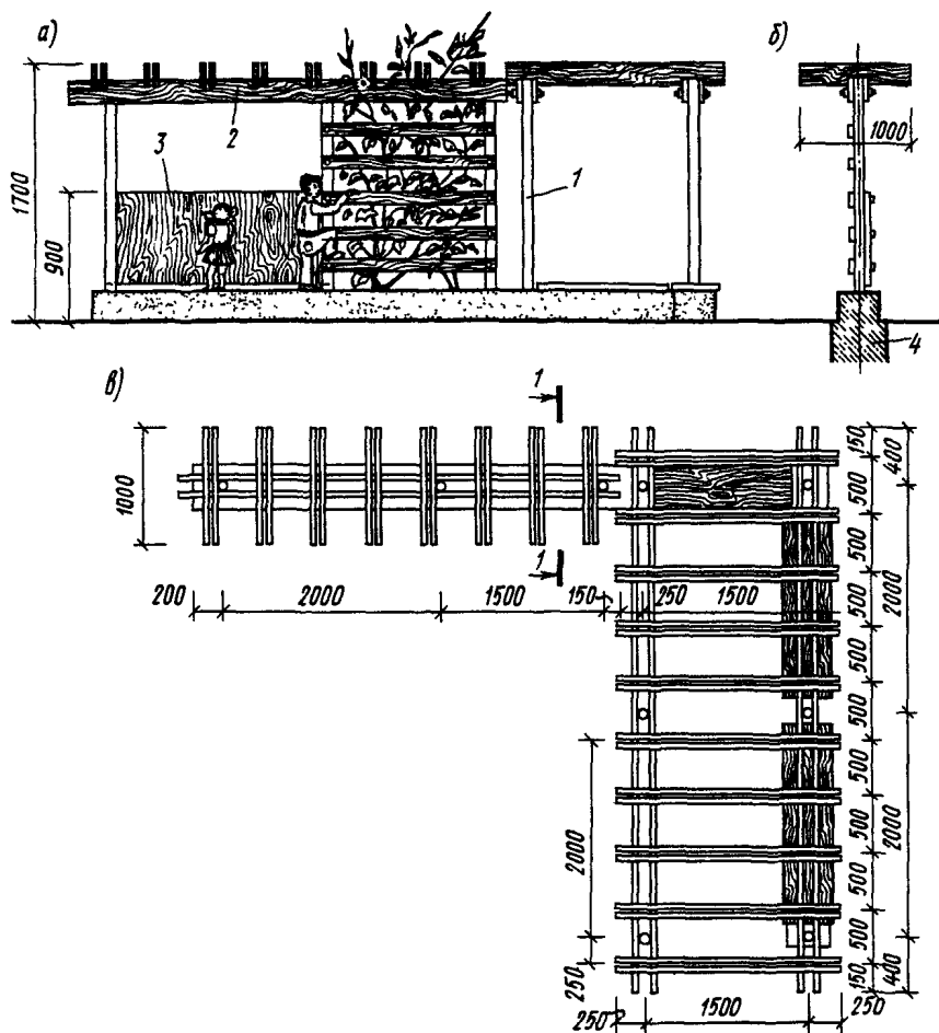
Рис. 21. Пергола на площадке дошкольного учреждения
