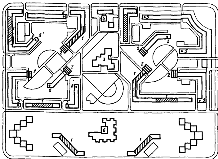
Рис. 3. Схема организации комплексов дошкольного воспитания в микрорайоне (ЦНИИЭП учебных зданий) 1 - встроенные в жилой дом помещения ясельных групп; 2 - пристроенные к торцам жилого дома помещения дошкольных групп (специализированного профиля); 3 - центр дошкольного воспитания с помещениями групп детского сада; 4 - предприятие централизованного обслуживания; 5 - помещения для групп кратковременного присмотра за дошкольниками; 6 - школа
