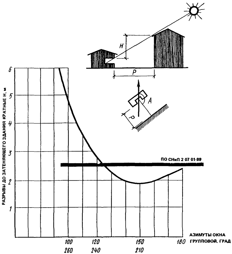
Рис. 9. График для определения величины разрыва между дошкольным учреждением и затеняющим объектом на равнине (ЦНТМОУ учебных зданий)
