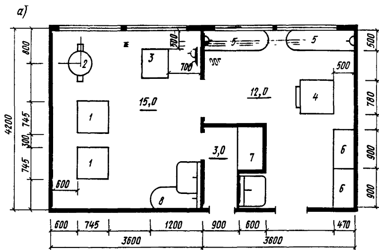
Рис. 50. Примеры планировок постирочных вместимостью а - свыше 150 до 250 мест; б - свыше 250 до 350 мест; 1 - машина стирально-отжимная автоматизированная с электро- обогревом; 2 - центрифуга для отжима выстиранного белья; 3 - котел или электрическое варочное устройство; 4 - бара- бан сушильный; 5 - стол гладильный; 6 - секция для белья; 7 - ларь для грязного белья; 8 - ванная для замачивания белья; 9 - пресс гладильный для сушки и глажения выстиран- ного и отжатого прямого и фасонного белья
