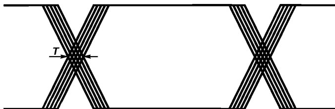
Рисунок 8 — Диаграмма, поясняющая измерение фазового дрожания цифрового сигнала
