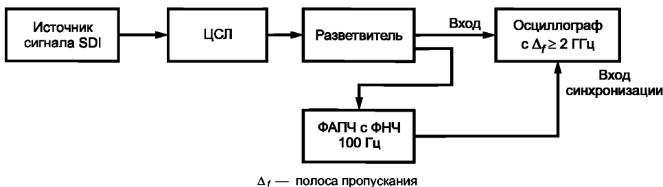
Рисунок 9 — Схема измерения высокочастотного фазового дрожания цифрового сигнала
