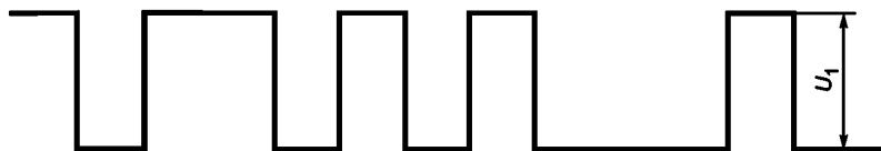
Рисунок 2 — Диаграмма, поясняющая измерение размаха сигнала
