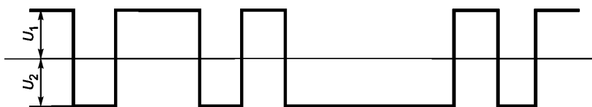
Рисунок 3 — Диаграмма, поясняющая измерение уровня постоянной составляющей
