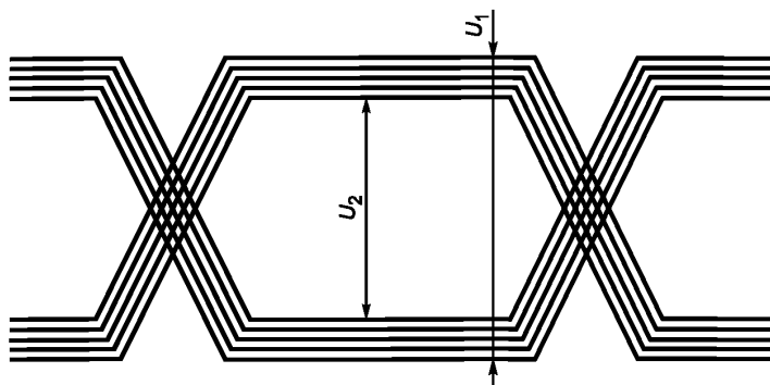
Рисунок 7 — Диаграмма, поясняющая измерение дрожания уровня цифрового сигнала
