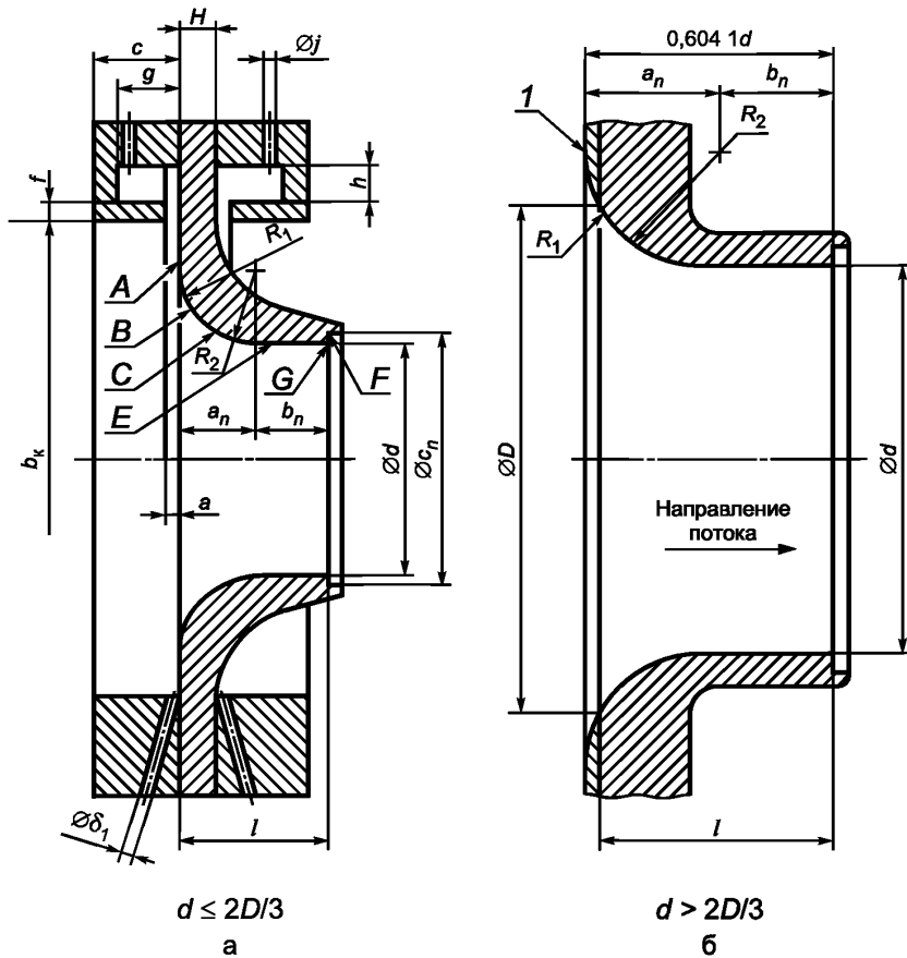
Рисунок 1 — Сопло ИСА 1932
