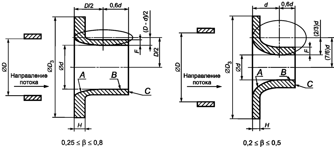
Рисунок 2 — Эллипсное сопло
