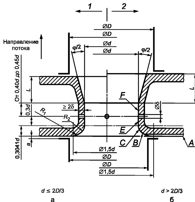
1 — укороченное сопло Вентури; 2 — неукороченное сопло Вентури
