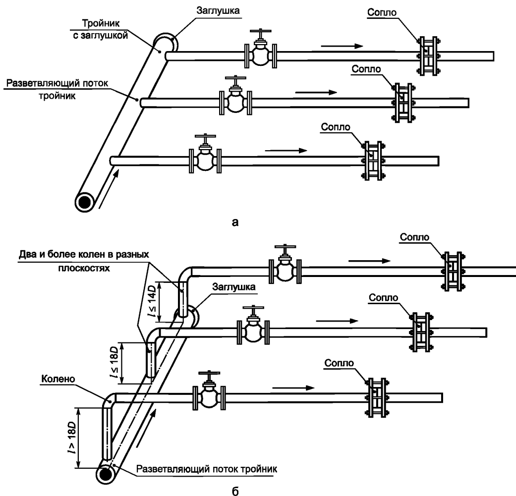
Рисунок 5 — Схемы коллектора
