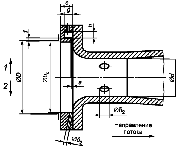
Рисунок 4 — Способы отбора давления, используемые для сопел Вентури
