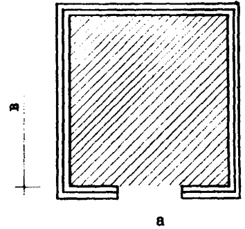
Минимальные параметры зоны хранения товаров в стационарной холодильной камере: a=2,4 a \times b \quad 6 \text{ м}^2
