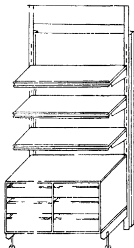
104 Горка пристенная с подшкафником с выдвижными ящиками Т03-37 длина 1022 ширина 687 высота 2245
