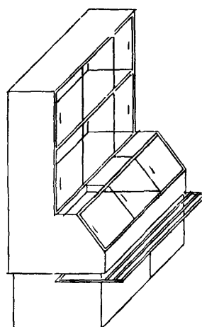
11 Прилавок-витрина 3-х ярусный охлаждаемый "ТАИР-132С" длина 1800 ширина 750 высота 1800
