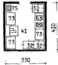
Помещение для подготовки мясо-рыбных товаров к продаже в универсаме "400"
