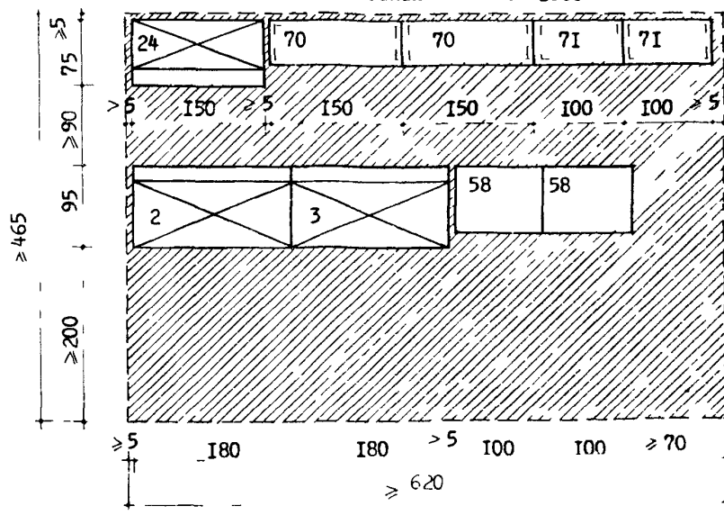
Зона хранения и выдачи заказов в универсамах торговой площадью 650 кв.м.
