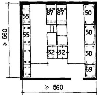
Кладовая овощей, фруктов, консервов и вина универсама "400"
