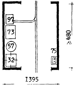
Помещение разрубочной в универсаме "1000"
