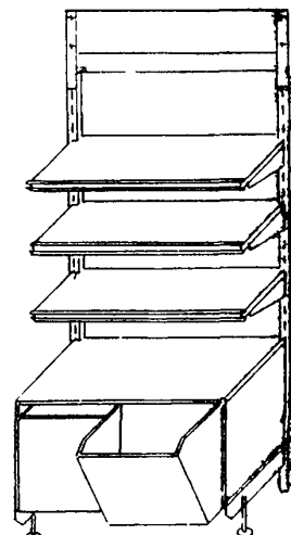
103 Горка пристенная с качающимися ларями Т03-32 длина 1022 ширина 687 высота 2245
