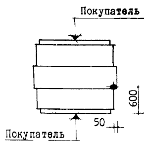
Витрина 2-х сторонняя 2-х ярусная неохлаждаемая "ТАИР-57"
