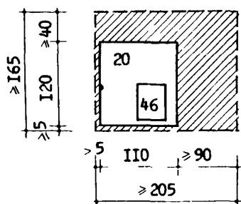
Зона рабочего места кассира и оплаты заказов
