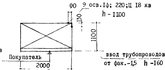
Прилавок-витрина для магазинов с продавцами ПВ-П
