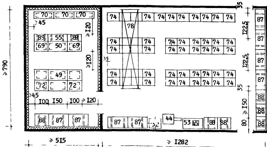
Кладовая овощей, фруктов и вино-водочных изделий универсама "1000"
