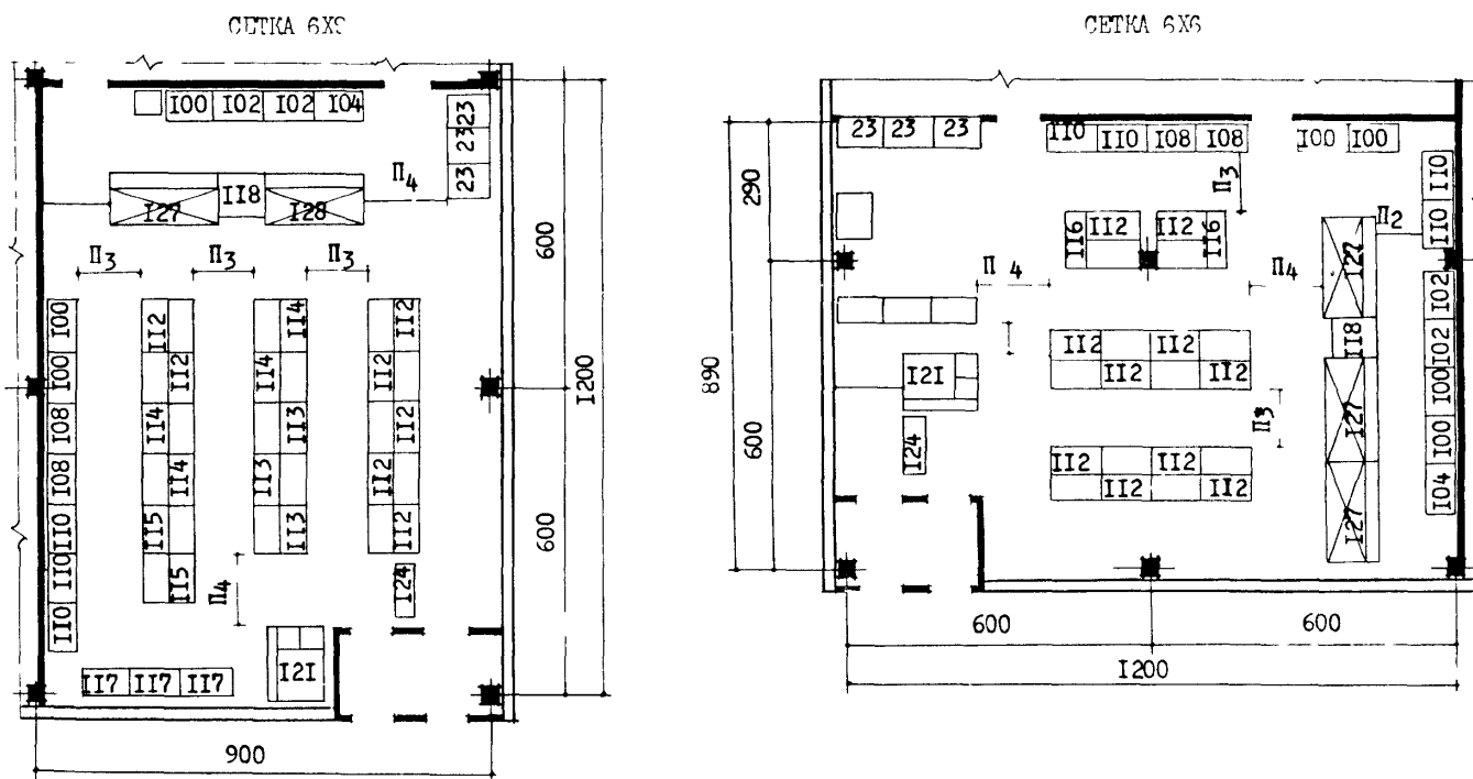
КОНСТРУКТИВНО-ПЛАНИРОВОЧНЫЕ СХЕМЫ УНИВЕРСАМА 100
