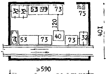
Помещение для подготовки к продаже рыбных товаров при условии фасовки и транспортирования товаров для отдела заказов в универсаме "1000"
