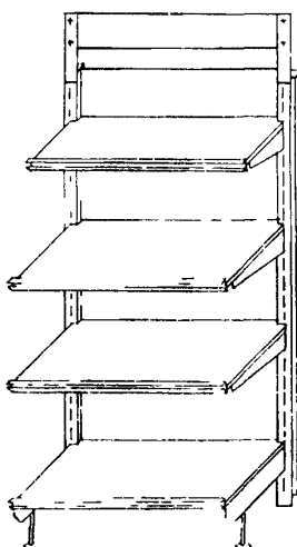
108 Горка пристенная для крупногабаритных товаров и тканей Т03-08 длина 1022 ширина 689
