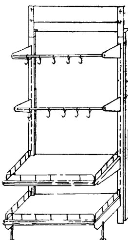
109 Горка пристенная для колбасных изделий Т03-36 длина 1022 ширина 689 высота 2245
