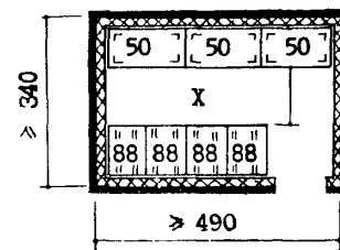
Охлаждаемая камера универсама "250"
