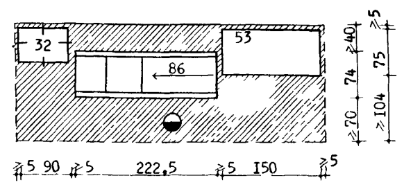
Зона упаковки гастрономических товаров под вакуумом
