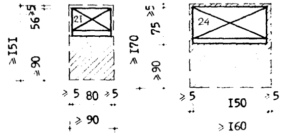
Зоны хранения товаров в холодильных шкафах типа ШХ-0,4 и ШХ-0,8
