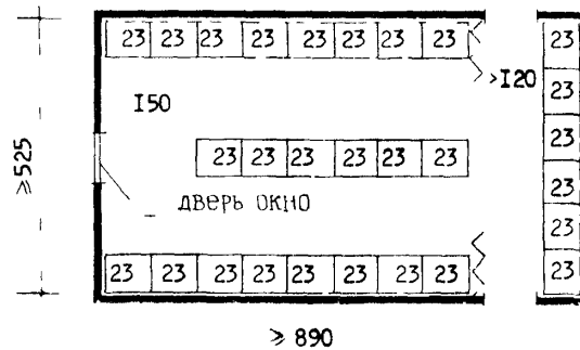
Кладовая хлебо-булочных изделий универсама "1000"
