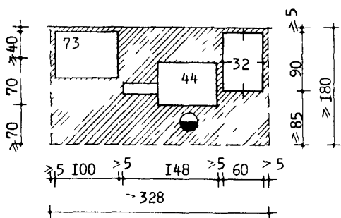
Зона упаковки овощей и фруктов в полиэтиленовую рукавную сетку
