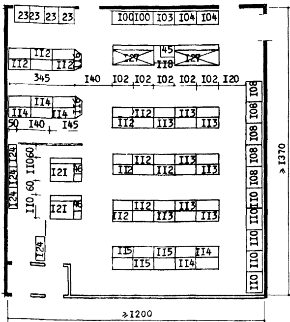
ГАБАРИТНЫЕ СХЕМЫ ТОРГОВОГО ЗАЛА УНИВЕРСАМА "150"
