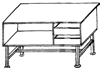
II20 Прилавок для отмеривания тканей Т03-16 длина 1417 ширина 802 высота 820
