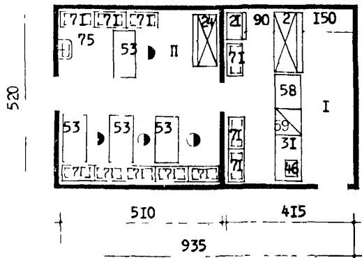
Отдел заказов на 2-х приемщиках при универсаме "400"
