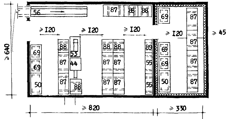
Кладовая овощей, фруктов и вино-водочных изделий универсама "650"
