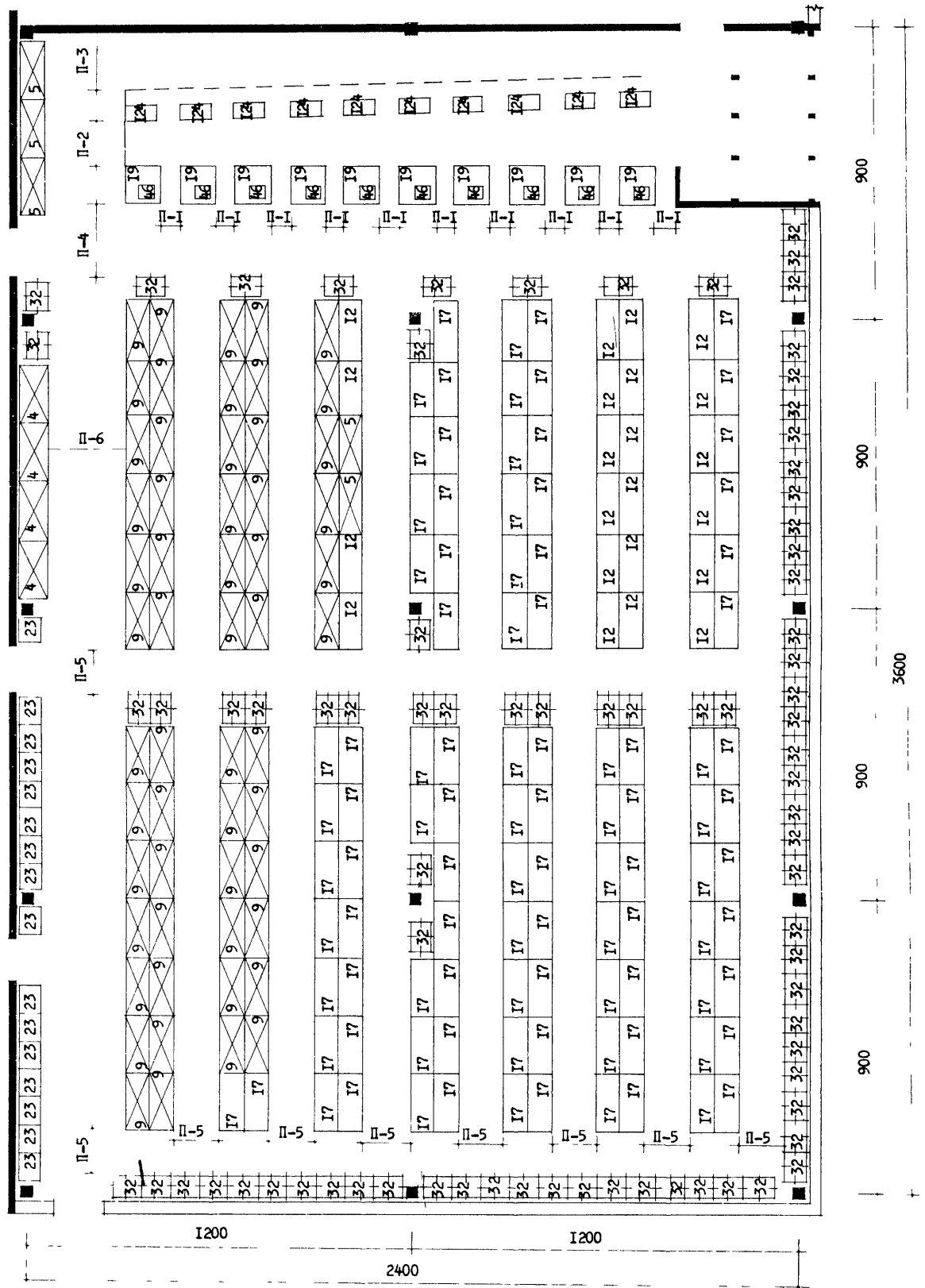
ТОРГОВЫЙ ЗАЛ УНИВЕРСАМА "ЮСО" "
