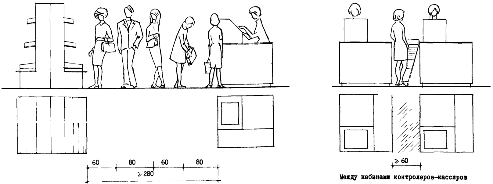
Между кабиной контролера-кассира и установленной параллельно ей горкой
