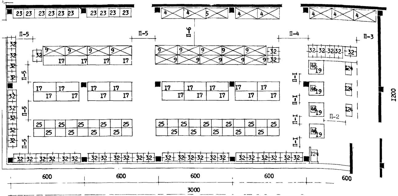
ТОРГОВЫЙ ЗАЛ УНИВЕРСАМА "650"
