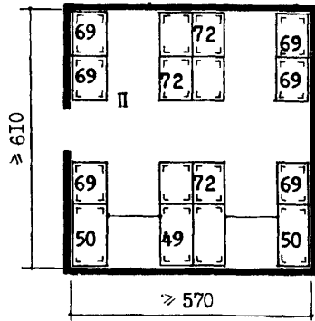
Кладовая продовольственных товаров универсама "250"
