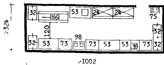
Помещение для подготовки к продаже гастрономических товаров в универсаме "1000"
