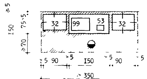
Зона взвешивания с одновременной фиксацией полного реквизита покупки предварительно расфасованных и упакованных продуктов на весах ВСК-3К
