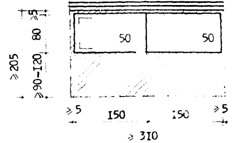
Зона хранения товаров на стеллажах в охлаждаемых камерах у стены без пристенной батареи-испарителя
