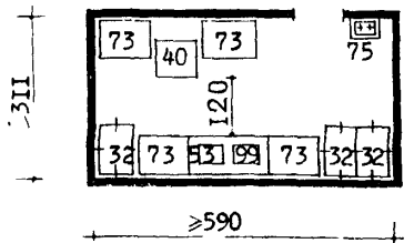
Помещение для подготовки к продаже рыбных товаров в универсаме "650"
