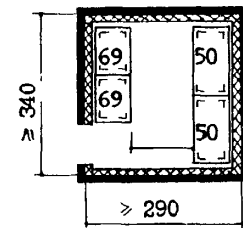
Охлаждаемая камера универсама "150"
