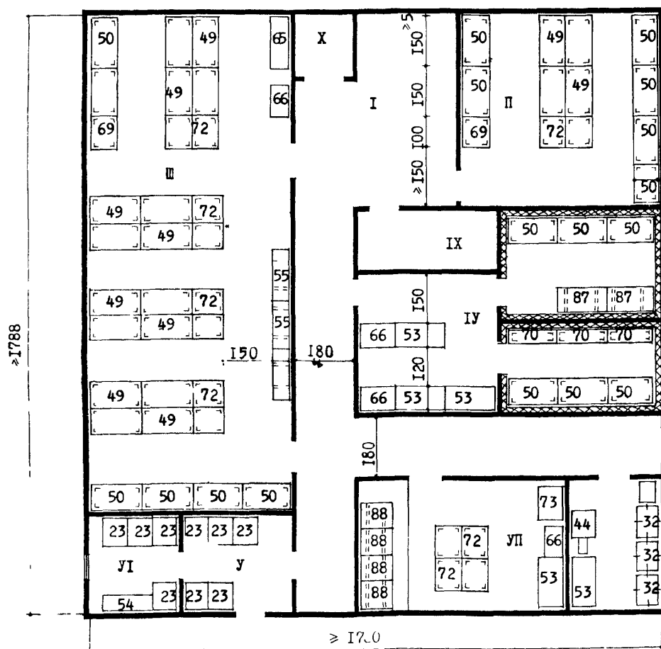
Планировочная схема помещения для приемки и хранения товаров универсама "400"
