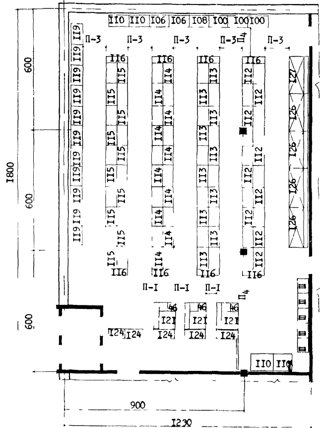
ТОРГОВЫЕ ЗАЛЫ УНИВЕРСАМА "250"
