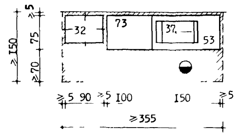
Зона резки монолитов сливочного масла на бруски
