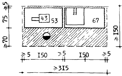
Зона приготовления мясного фарша на мясорубке типа МИП-82
