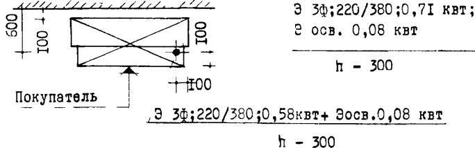
Прилавок-витрина 3-х ярусный охлаждаемый "ТАИР-132"
