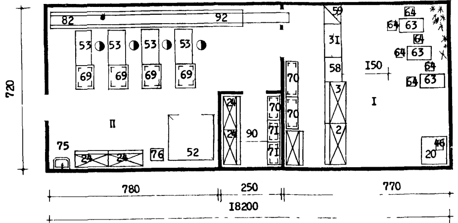
Отдел заказов на 3-х приемщиках при универсаме "650"
