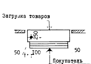
Трилавок-витрина 3-х ярусный неохлаждаемый "ТАИР-351"
