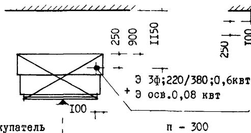
Прилавок-витрина охлаждаемый "ТАИР-106"
