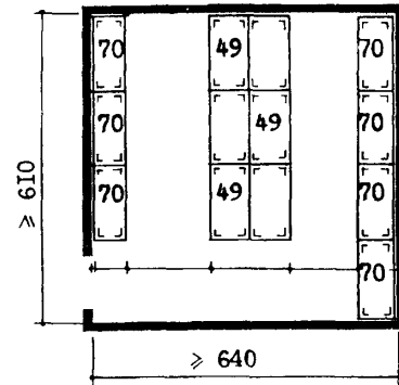
Кладовая бакалейных и кондитерских товаров универсама "400"
