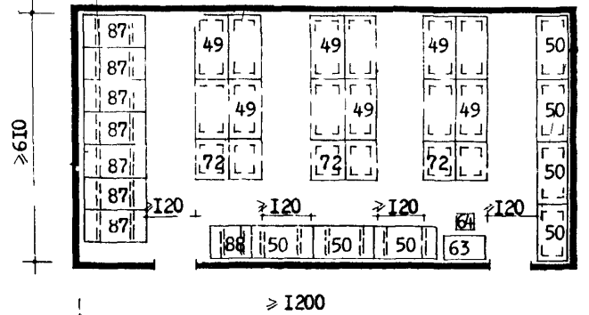
Кладовая непродовольственных товаров универсама "400"
