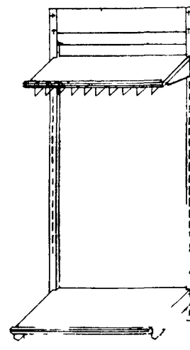
107 Горка пристенная с выдвижными штангами для полок, коробок, тканей и т.д. Т03-38 длина 1022 ширина 689 высота 2245
