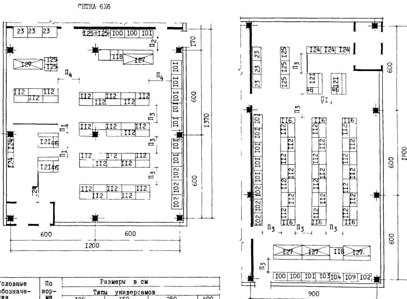
КОНСТРУКТИВНО-ПЛАНИРОВОЧНЫЕ СХЕМЫ УНИВЕРСАМА 150
