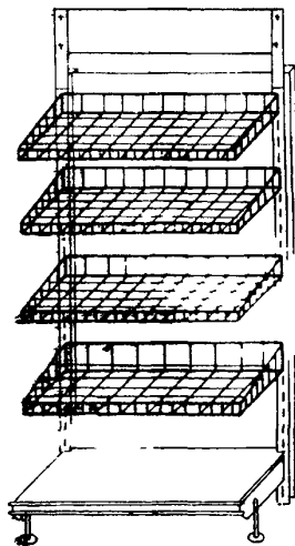
102 Горка пристенная с корзинами Т03-02 длина 1022 ширина 689 высота 2245
