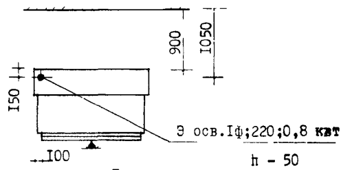
Прилавок-витрина неохлаждаемый "ТАИР-305"
