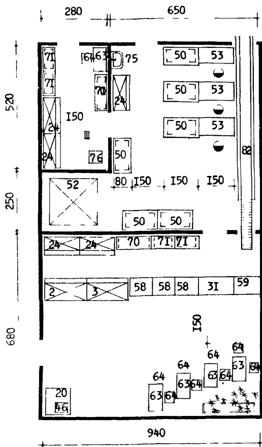
Отдел заказов на 4-х приемщиках при универсаме "400"
