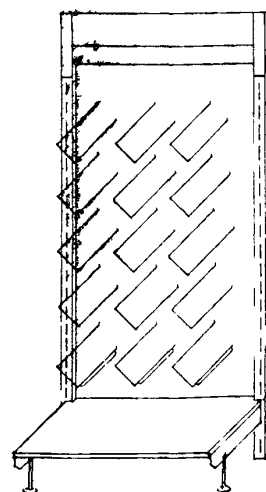
110 Горка пристенная для обуви Т03-11 длина 1022 ширина 689 высота 2245
