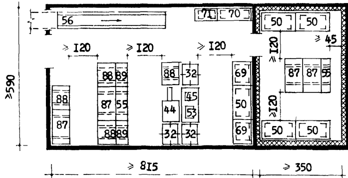
Кладовая овощей, фруктов и вино-водочных изделий универсама "400"
