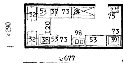
Помещения для подготовки к продаже молочно-жировых и гастрономических товаров в универсамах "400" и "650"
