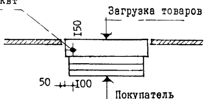
Прилавок-витрина неохлаждаемый "ТАИР-345С"
