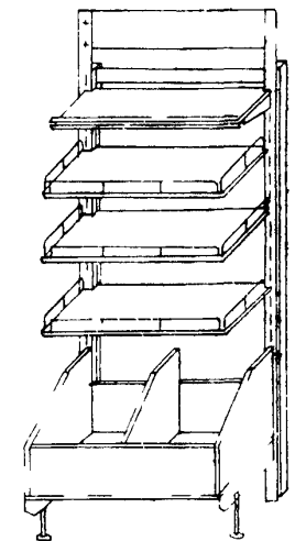
111 Горка пристенная для хлеба Т03-12 длина 1022 ширина 689 высота 2245
