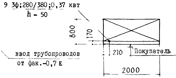
Прилавок-витрина охлаждаемый ПВ-СМ
