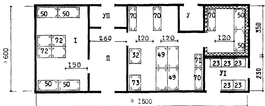
Планировочная схема помещений для приемки и хранения товаров универсама "100"
