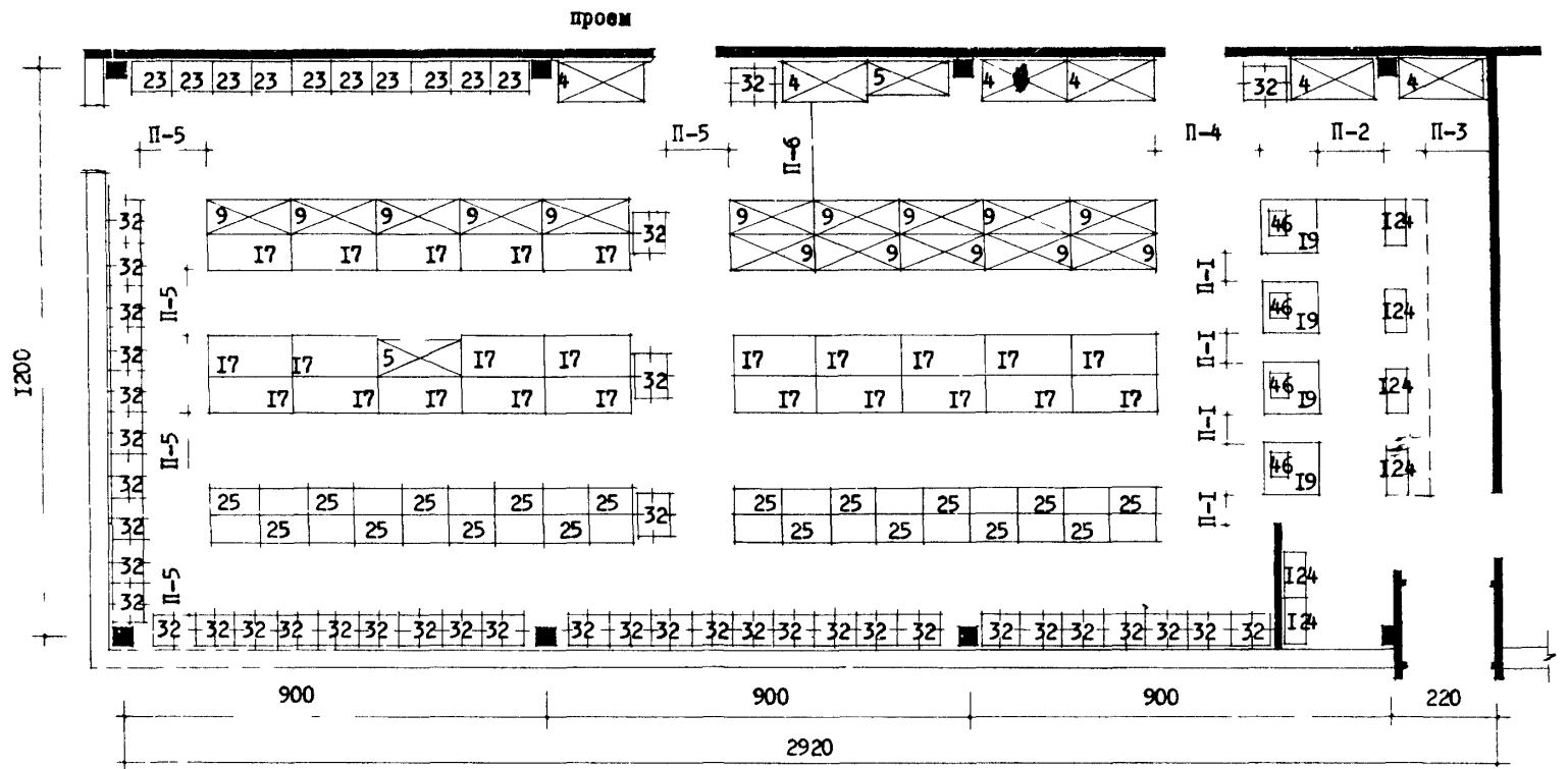
ТОРГОВЫЙ ЗАЛ УНИВЕРСАМА "650"
