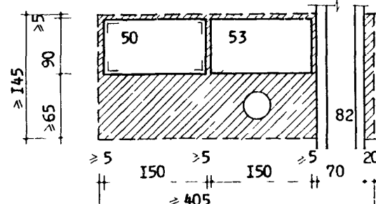
Зона рабочего места фасовщика и контролера-упаковщика в универсамах "650" и "1000"
