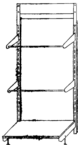
106 Горка пристенная для одежды Т03-40 длина 1022 ширина 689 высота 2245
