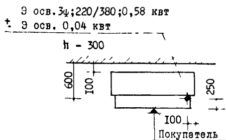
Витрина пристенная над наклонным подъемником "ТАИР-29"
