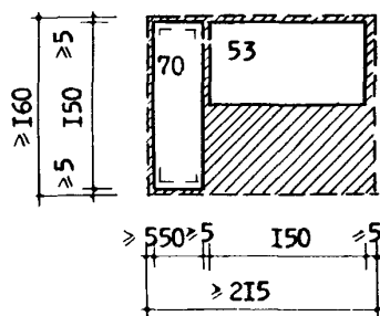
Зона рабочего места фасовщика и контролера-упаковщика в универсамах "400"
