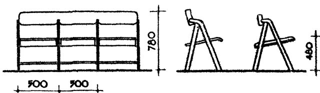
11) СЕКЦИЯ СКЛАДНЫХ СТУЛЬЕВ
