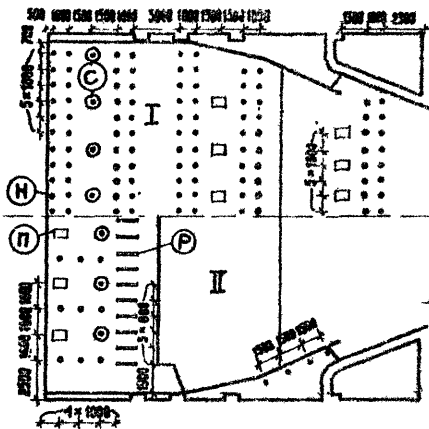
И - ПЛАН РАЗЕДКИ СВЕТИЛЬНИКОВ НАД ЗАЛОМ
