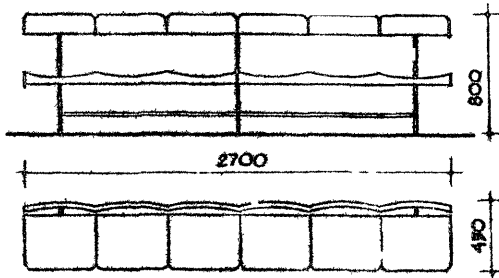
9) СКАМЬЯ СКЛАДЫВАЮЩАЯСЯ
