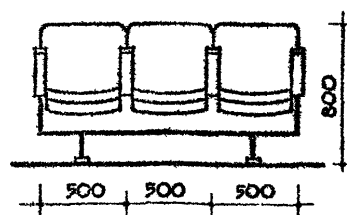
4 КРЕСЛО ПОЛУМЯГКОЕ, КАРКАС МЕТАЛЛИЧЕСКИЙ
