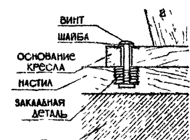
г. КРЕПЛЕНИЕ КРЕСЛА К ДЕРЕВЯННОМУ ПОЛУ ПРИ ПОМОЩИ ЗАКЛАДНОЙ ДЕТАЛИ.
