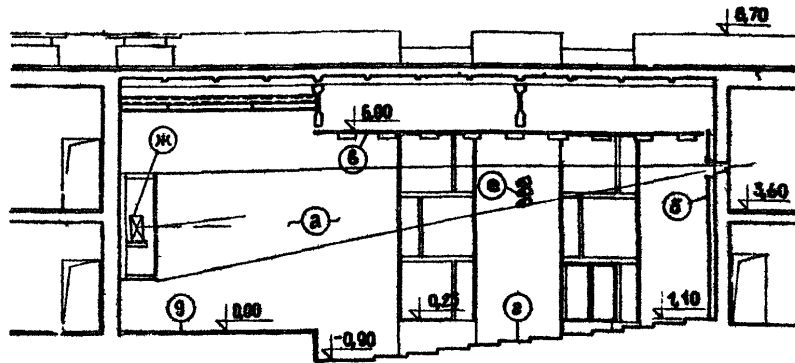
РАЗРЕЗ по А-А
