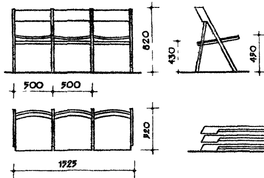
11) СЕКЦИЯ СКЛАДНЫХ СТУЛЬЕВ
