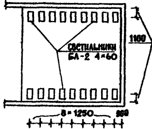
ПЛАН РАЗБИВКИ СВЕТИЛЬНИКОВ
