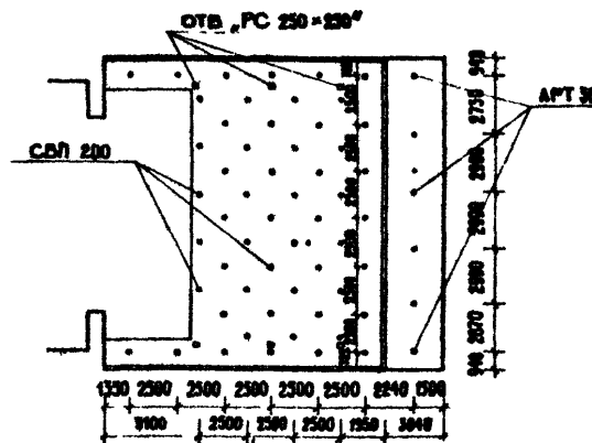
ПЛАН РАЗБИВКИ СВЕТИЛЬНИКОВ
