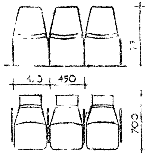
7) КРЕСЛО С ПОПЛИТРОМ СКЛАДИРУЕМОЕ
