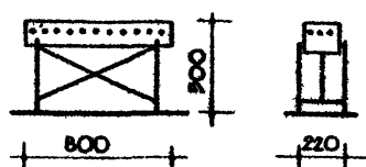
19 ПОДСТАВКА ДЛЯ КИНОПРОЕКТОРА
