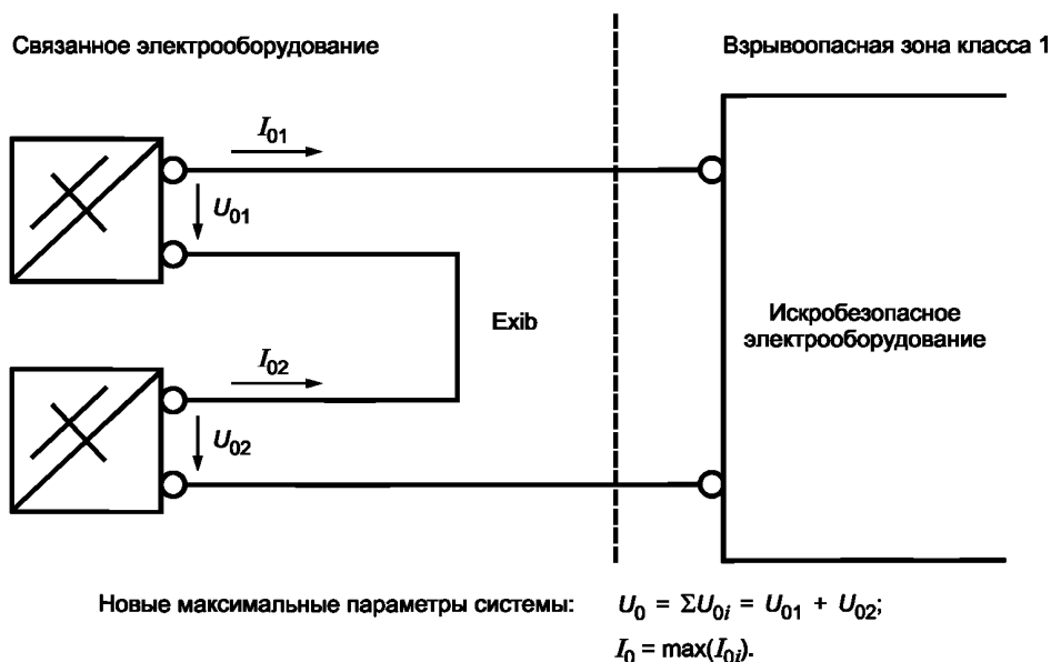
Рисунок В.1 — Последовательное соединение. Суммирование напряжений
