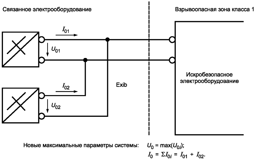
Рисунок В.2 — Параллельное соединение. Суммирование токов
