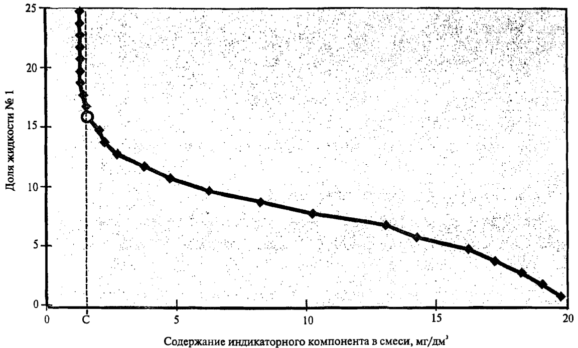
Рисунок 8.2 – График смешения жидкостей
