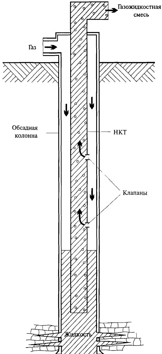
Рисунок 17.1 – Газлифт
