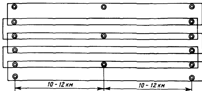
Рис. 5. Съемка в мащабта 1:10 000 с сечением рельефа чрез 5,0 м
