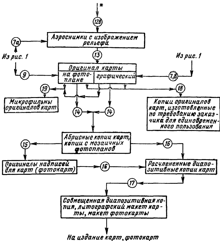
Рис. 2. Технологическая схема камеральных работ при стереотопографической съемке в масштабах 1:10 000 и 1:25 000 (съемка рельефа на топографическом стереометре СТД-2 и составление оригиналов карт на фотопланах, пластике или основе).
