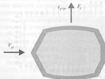
Рисунок 4.4. Определение критических скоростей ветра и аэродинамических сил при резонансном вихревом возбуждении
