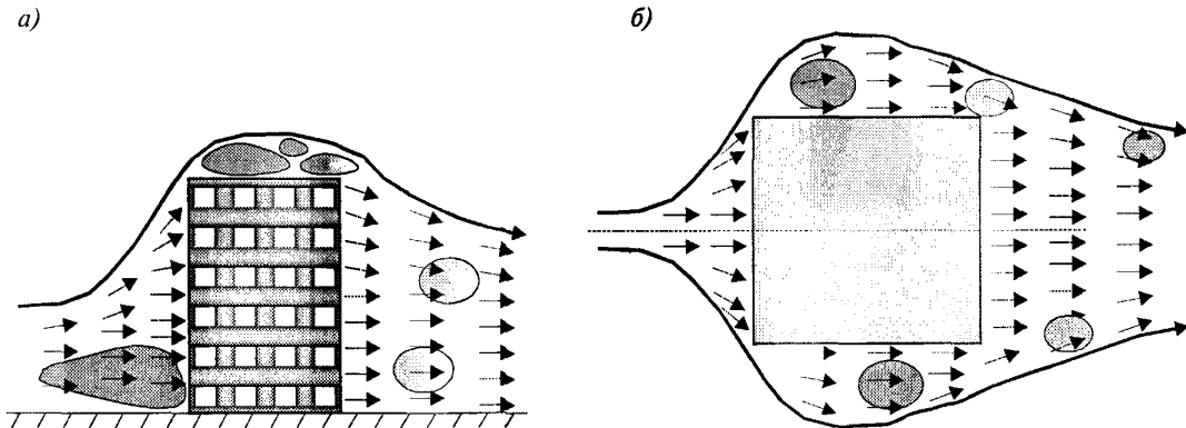
Рисунок 4.1. Качественная картина обтекания здания
