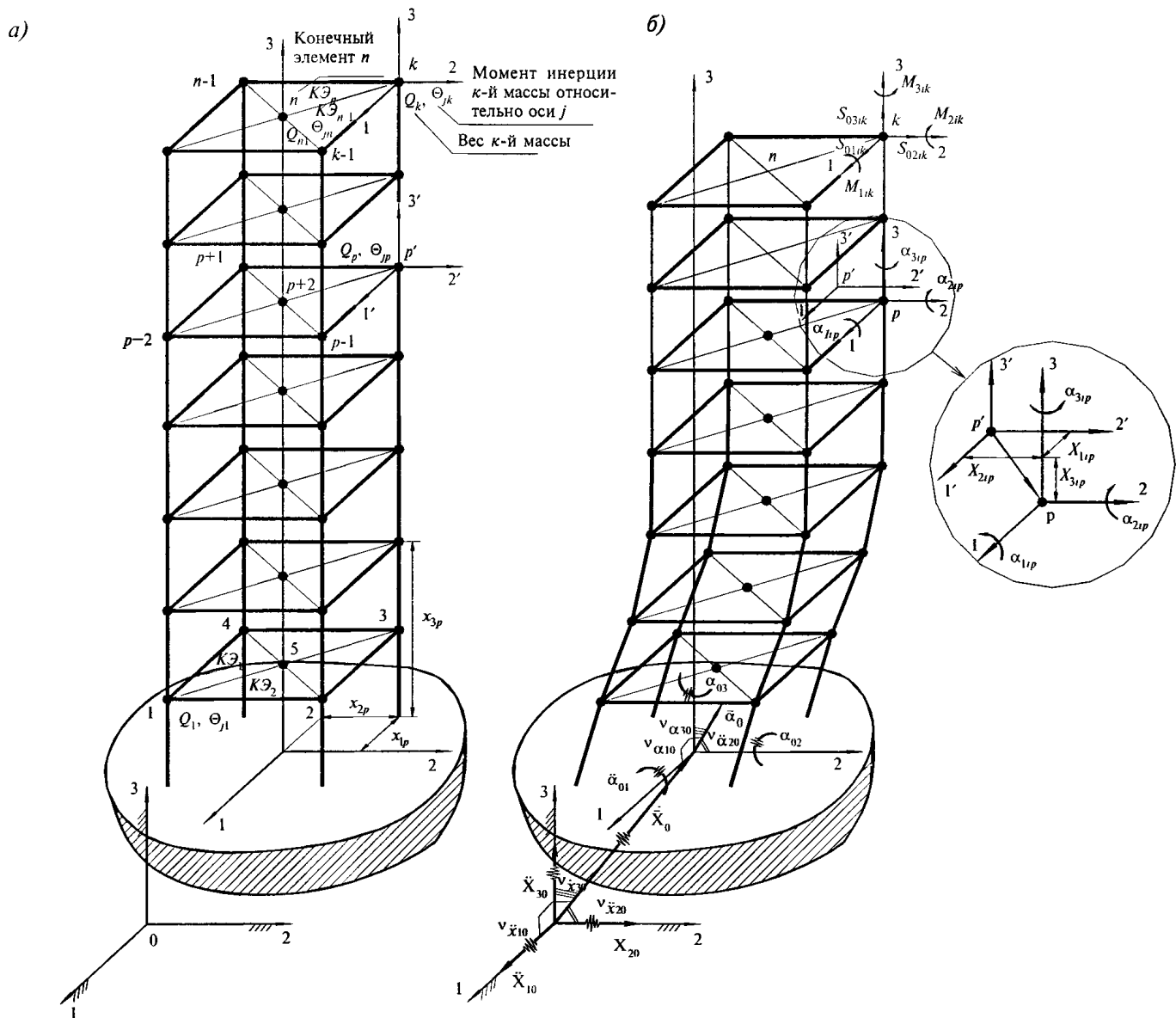
Рисунок 7.5. Пространственная расчетная динамическая модель сооружения при интегральной модели сейсмического воздействия
