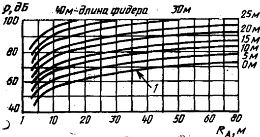
Зависимость затухания электромагнитных волн в свободном пространстве и в фидере РК 75—13—17 для частот 1535— 1543,5 МГц от расстояния между антеннами и длины фидера
