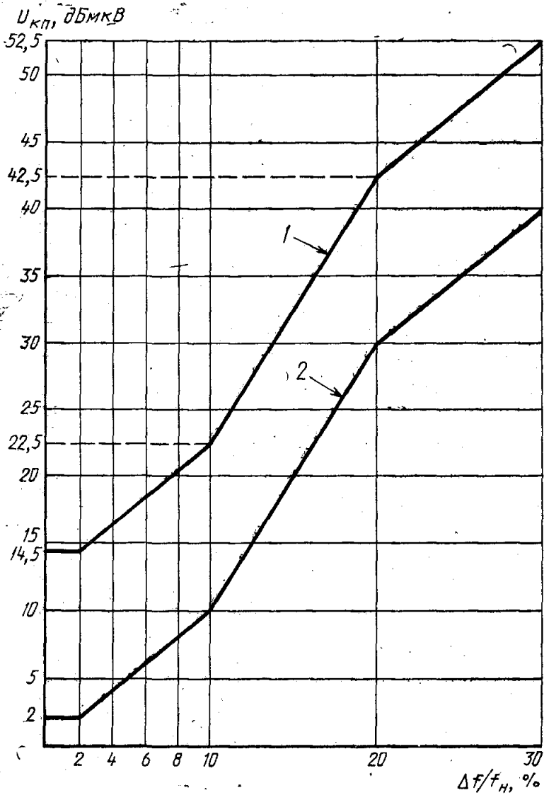
1 — при расстоянии 10 м от приемной антенны; 2 — при расстоянии 3 м от приемной антенны; f_n — частота настройки радиопередатчика; \Delta f — частота отстройки радиоприемника от частоты настройки радиопередатчика
