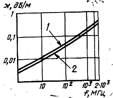
Зависимость потерь в фидере РК 75—13—17 от частоты
