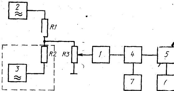
Структурная схема измерения внеполосных излучений радиопередатчиков, работающих в режиме ЗЭЕ
