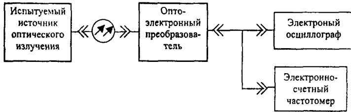
Рисунок 4 - Схема измерения амплитудно-временных параметров импульсно-модулированного сигнала
