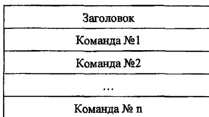
Рисунок 8.1 - Формат пакета SCTP
