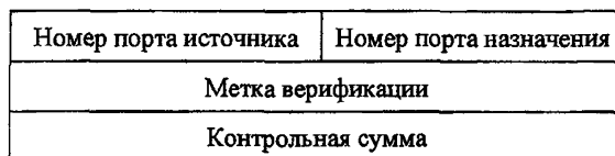
Рисунок 8.2 - Формат заголовка пакета SCTP
