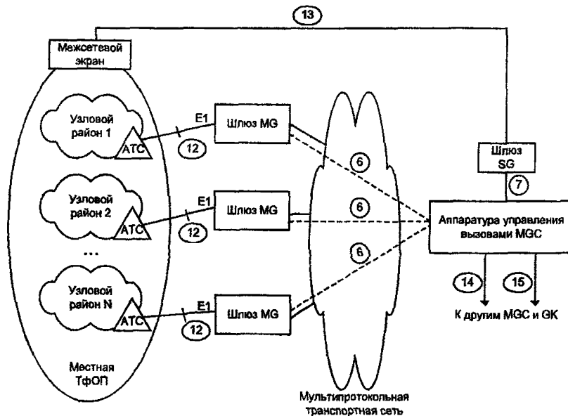
Рисунок 5.2 – Схема организации транзитной станции коммутации
