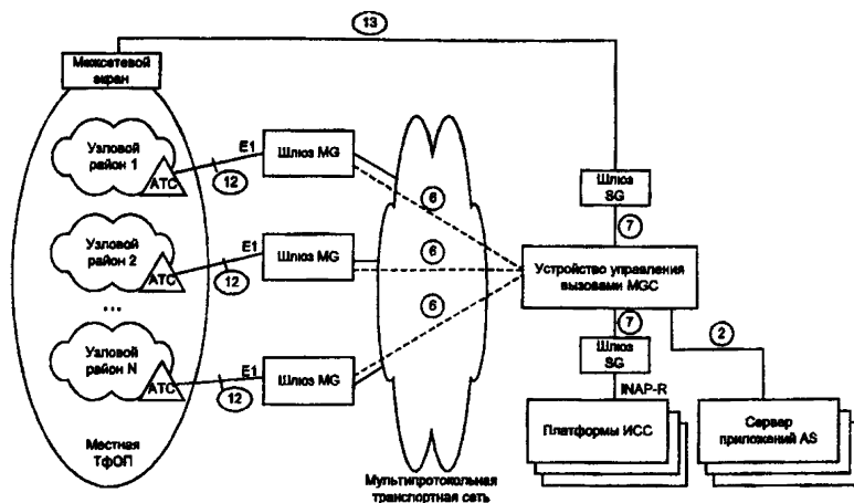
Рисунок 5.3 – Схема организации распределенного SSP
