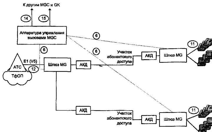
Рисунок 5.1 – Схема организации распределенного телефонного концентратора
