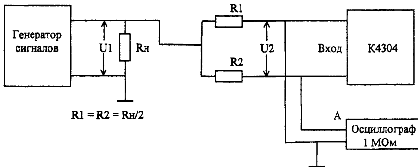
Рисунок 6.6 Измерение затухания асимметрии входа прибора
