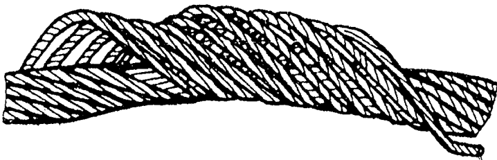
Рис. 15. Корзинообразная деформация
