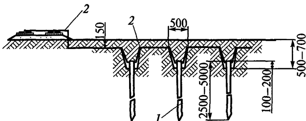
Рис. 13. Схема соединения вертикальных заземлителей: 1 — заземлитель; 2 — заземляющий проводник
