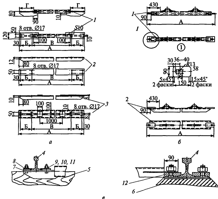
Рис. 9. Конструкции стяжек:
