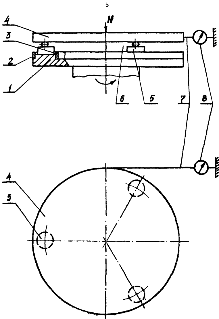
Рис.1. Схема испытательной установки /рабочего узла/
