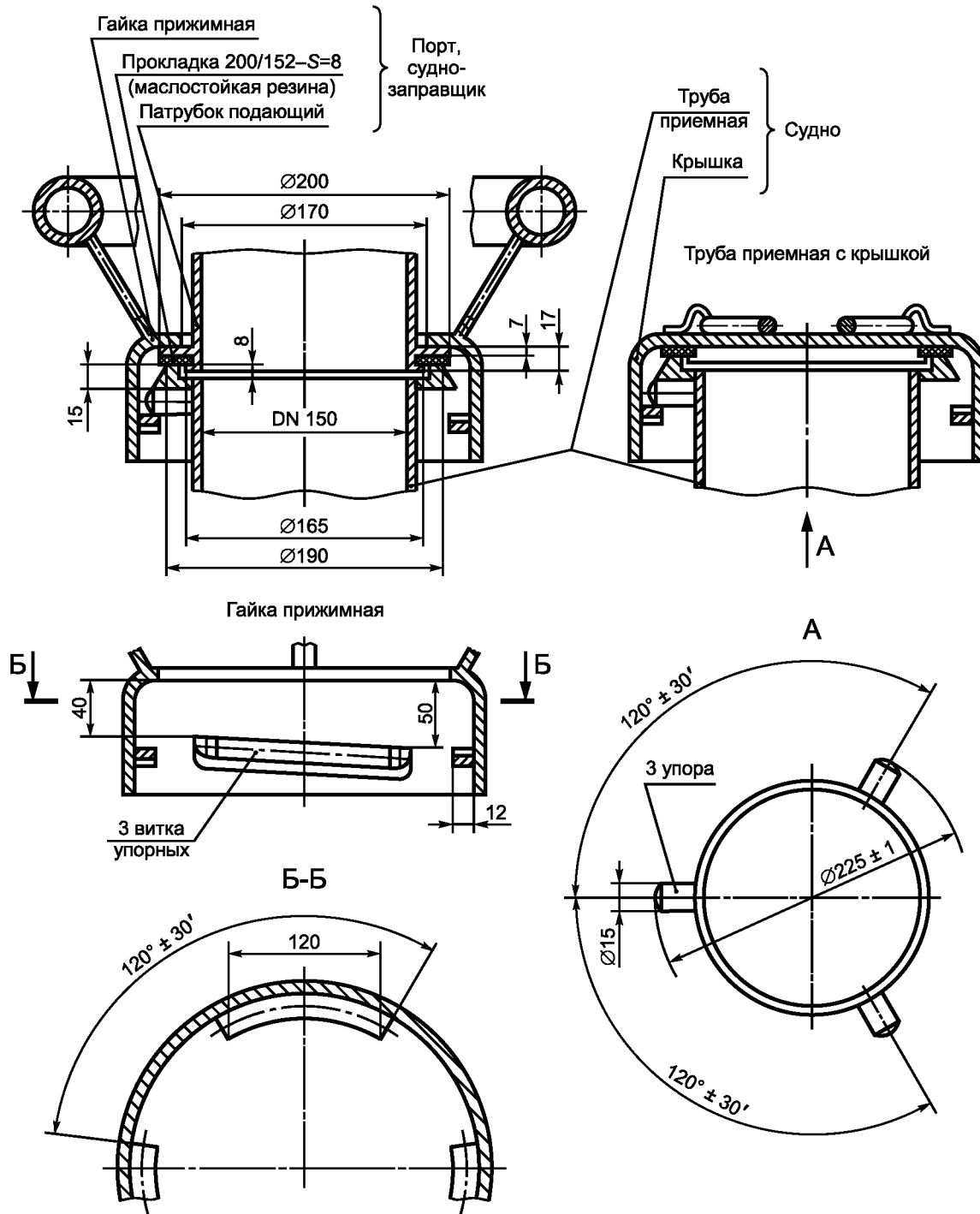
Рисунок 2 — Устройство для приема топлива номинальным диаметром 150 мм
