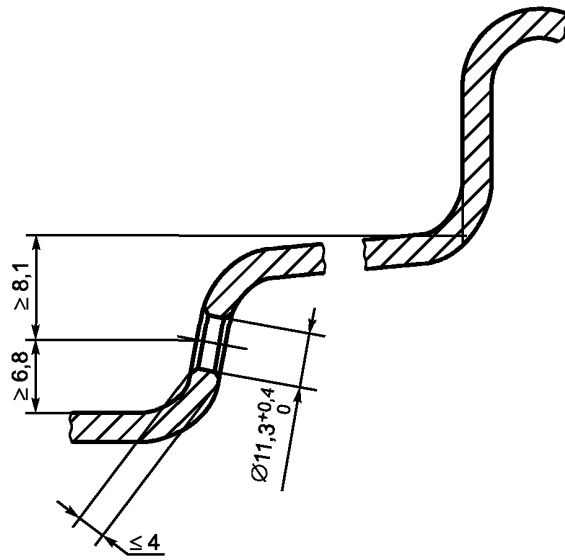
Рисунок 3 — Размеры вентиляционного отверстия для бескамерных шин
