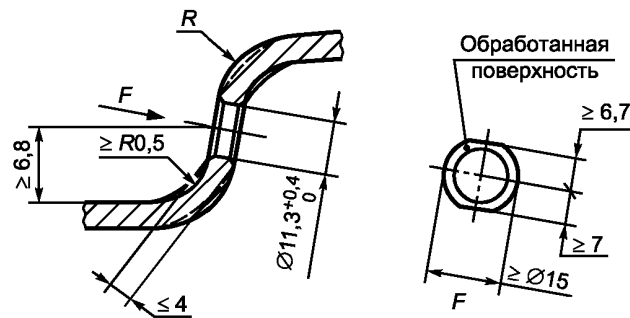
Рисунок 4 — Исполнение поверхности в зоне вентиляционного отверстия
