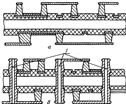
1 — металлизированные отверстия
