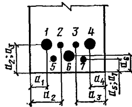
Рис. 2. Среднее расстояние до осей арматуры
