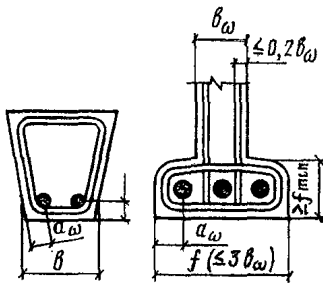
Рис. 3. Армирование балок и расстояния до оси арматуры
