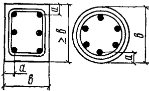
Рис. 1. Расстояния до оси арматуры
