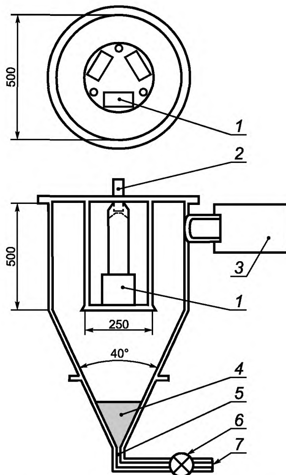
1 — втягивающее устройство; 2 — механизм управления циклами; 3 — пылеуловитель; 4 — пыль; 5 — фильера; 6 — кран и фильтр; 7 — воздух
