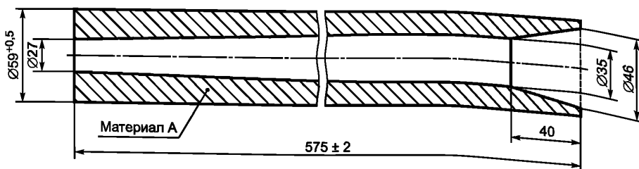
Рисунок Е.12 — Полиуретановая трубка
