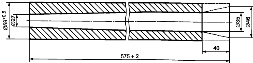
Рисунок Е.7 — Полиуретановая трубка из материала А
