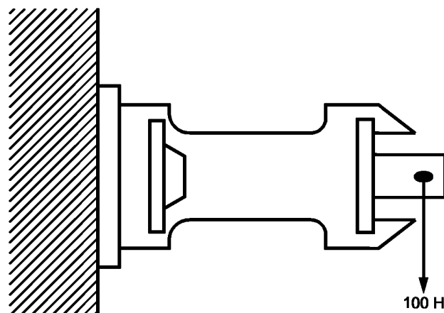
Рисунок И.16 — Монтаж элемента шеи в комплекте
