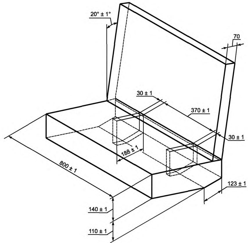
Рисунок E.5 — Размеры сиденья (трехмерное изображение)
