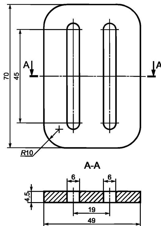
Рисунок П.3 — Центральная деталь стандартного ремня безопасности
