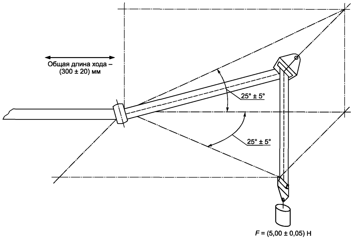
Рисунок Д.4 — Испытание с направляющим устройством
