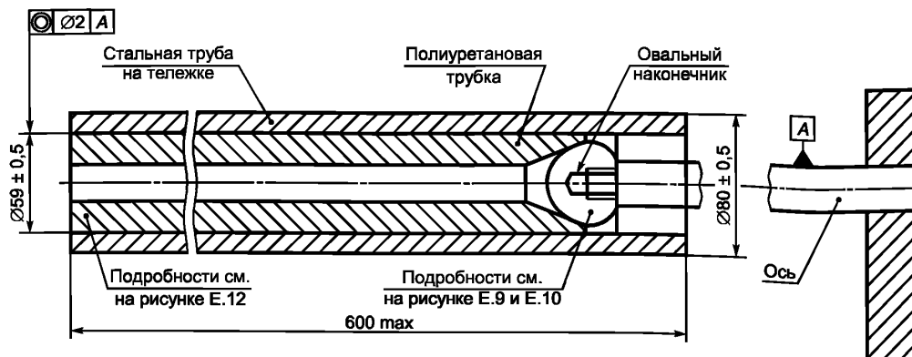
Рисунок Е.11 — Стопорное устройство в сборе
