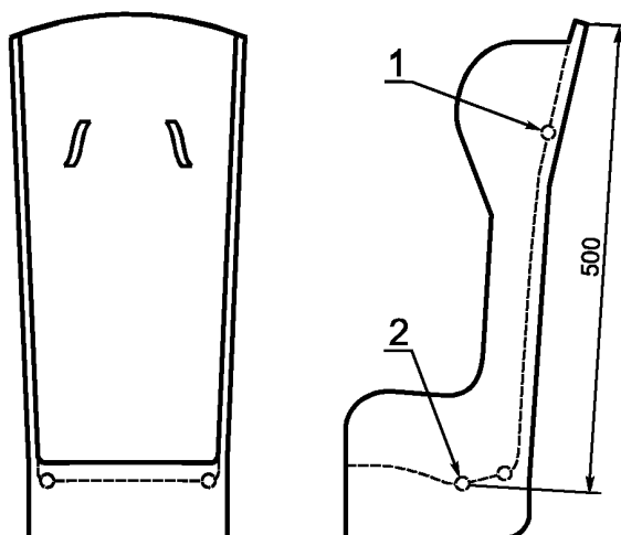
Рисунок Н.1 — Места крепления
