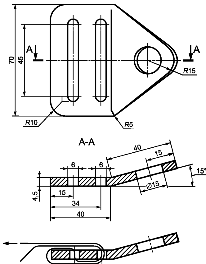
Рисунок П.2 — Стандартная пластина для крепления
