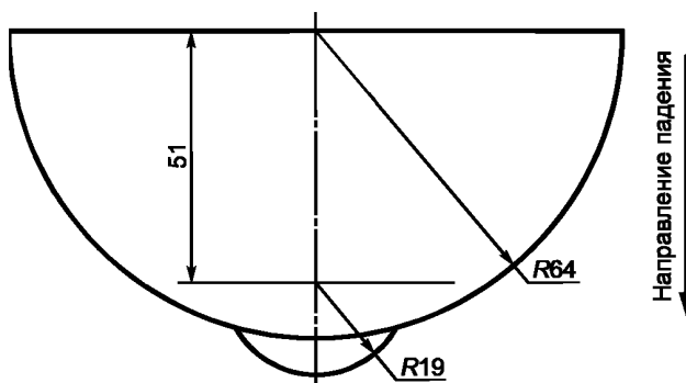
Рисунок Т.1 — Модель головы
