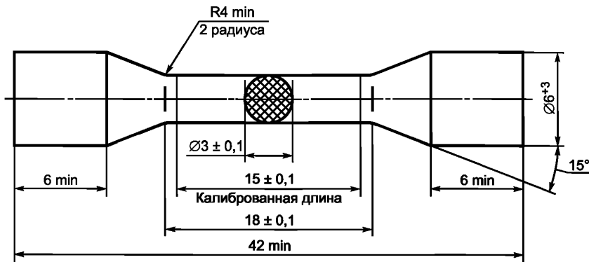
Рисунок 1 — Образец с короткой головкой
