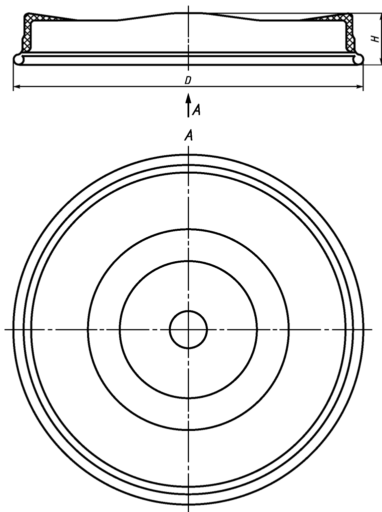
Рисунок Б.1 — Крышка ПТ
