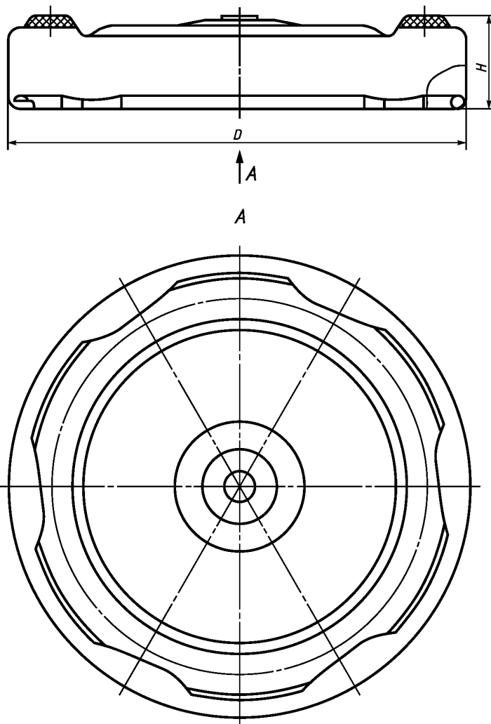
Рисунок А.4 — Крышка RSB
