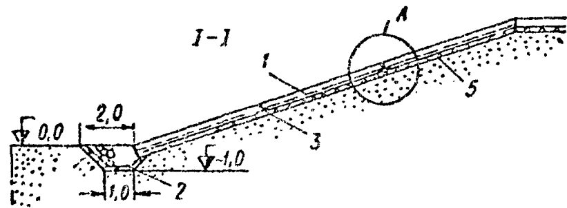
Рис. 7. Схема крепления монолитными железобетонными плитами: 1—плиты; 2—упорная каменная призма, уложенная на слой щебня; 3—балочки; 4—швы; 5—слой щебня (гравия); 6—битумный мат; 7—деревянная доска; 8—арматурная сетка
