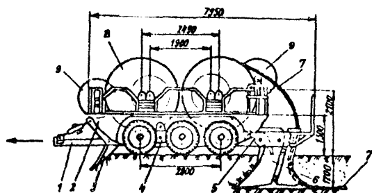
рис. 6 Кабелеукладчик КВ-К-3
