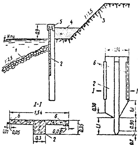
Рис. 10 Крепление откосов вертикальными стелками из железобетонного шпунта.
