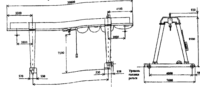
Пролет 13,0 м
