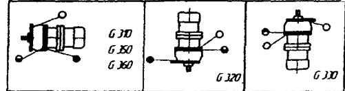
Motor-редуктор на опорном фланце
