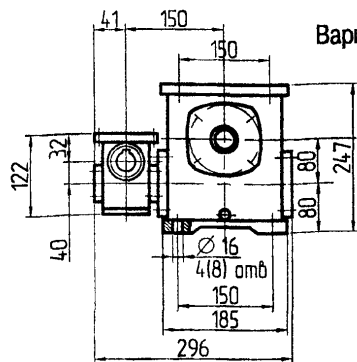
Вариант крепления 1 (2)
