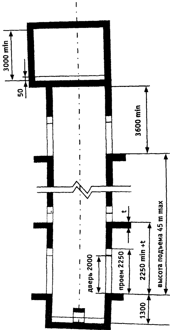
Разрез шахты
