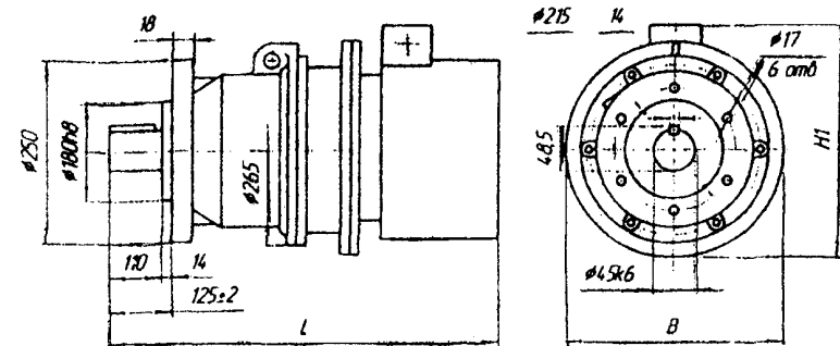
Мотор-редуктор фланцевое исполнение
