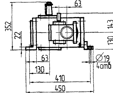
Вариант сборки 51, вариант крепления 3
