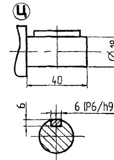
Варианты исполнения концов быстрого вала
