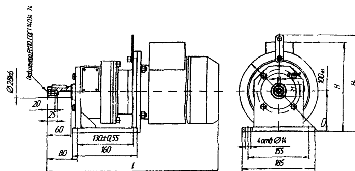
Мотор-редуктор на лапах
