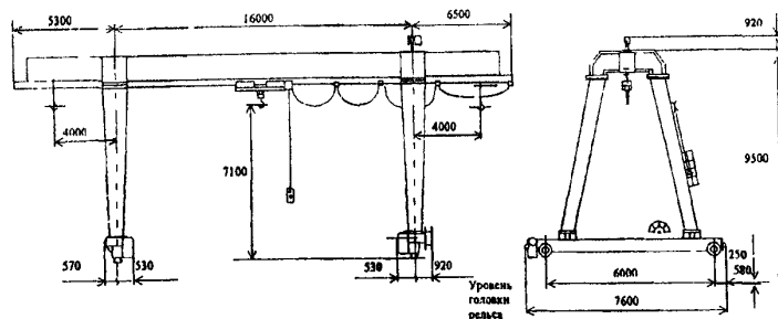
Пролет 16,0 м
