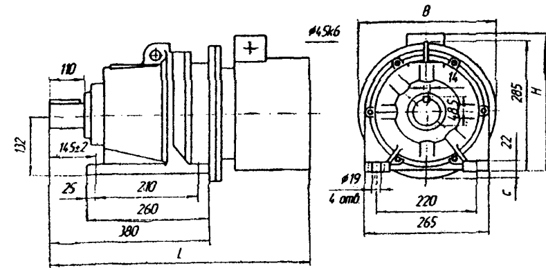
Мотор-редуктор на лапах
