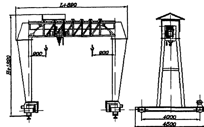
Кран г/п 5,0 т
