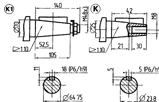
Вариант сборки 51 (53) Вариант крепления 1 (2)
