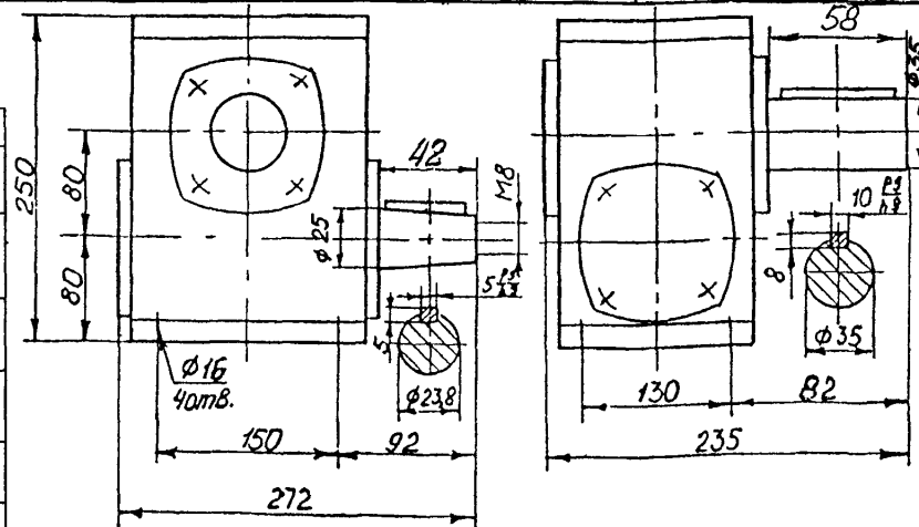
Варианты сборки:
