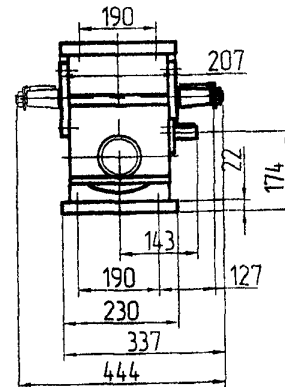
Вариант сборки 51 (53) Вариант крепления 1 (2)
