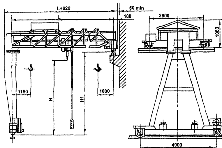
Краны г/п 3, 2 т
