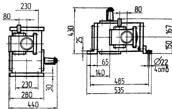
Вариант сборки 51, вариант крепления 3
