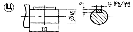
Варианты исполнения концов тихоходного вала
