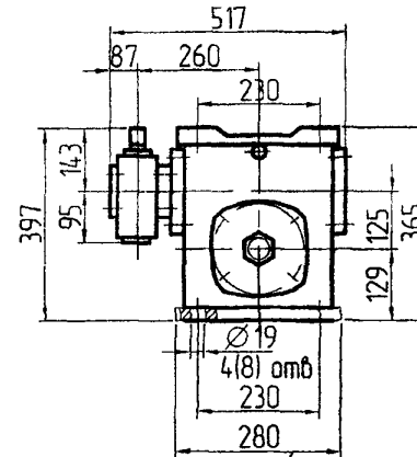
Вариант сборки 52, вариант крепления 1 (2)
