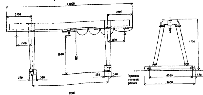
Пролет 13,0 м
