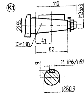
Варианты исполнения концов тихоходного вала
