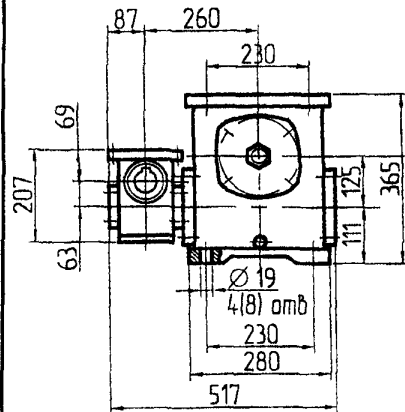
Вариант сборки 51 (53) Вариант крепления 1 (2)
