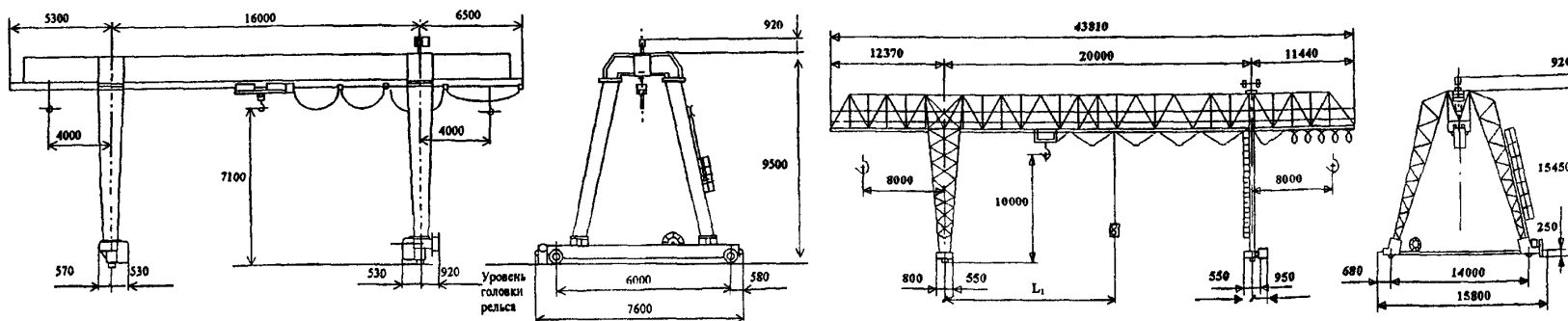
Краны г/п 10 т
