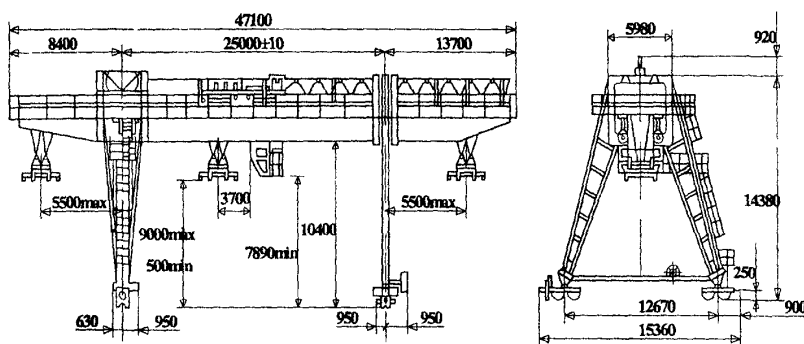
КК24.00.00.000 ГЧ
