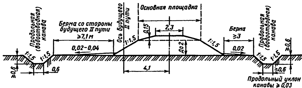
Рис. П.3.3. Насыпи высотой до 2 м
