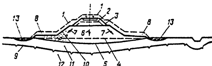
Рис. П.8.22. Осадки и расползание насыпи на оттаивающих вечномерзлых грунтах:
