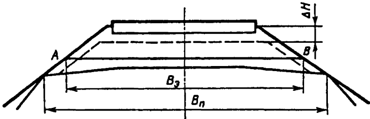
Рис. П.5.3. Построечное и эксплуатационное очертания основной площадки земляного полотна из глинистых грунтов после проведенной подъемки пути на величину \Delta H для компенсации оседания земляного полотна, при неизменном типе верхнего строения пути или после подъемки пути на балластные материалы (против построечного положения):
