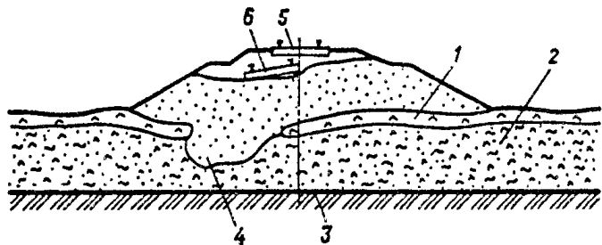
Рис. П.8.30. Провалы насыпей на торфяных болотах (илистых отложениях):
