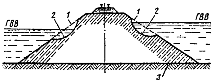
Рис. П.8.39. Размывы подтопляемых откосов земляного полотна: 1 — построчный откос насыпи; 2 — место размыва; 3 — основание насыпи
