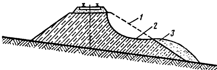
Рис. П.8.14. Оползание откосов насыпи:
