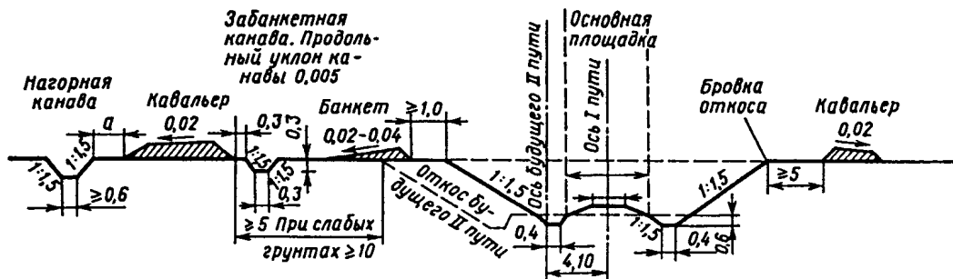
Рис. П.3.1. Выемки глубиной до 12 м
