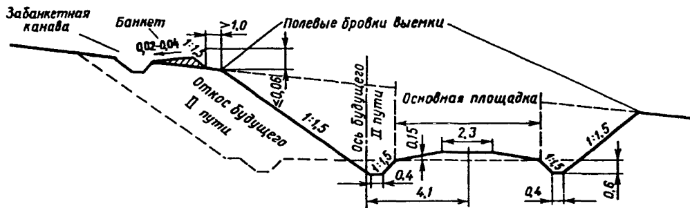
Рис. П.3.2. Выемки на косогорах
