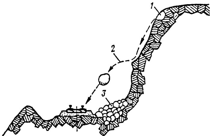
Рис. П.8.18. Вывалы:
