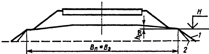
Рис. П.5.1. Типовое (построечное) очертание основной площадки однопутного земляного полотна из глинистых грунтов с шириной B_n , расположением бровки на отметке H и высотой сливной призмы h_{сп} ; 1 — откос насыпи; 2 — откос кювета в выемке
