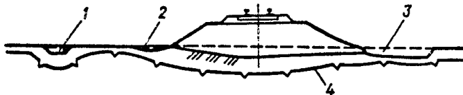
Рис. П.8.5. Термокарстовые понижения и провалы на мари и земляном полотне:
