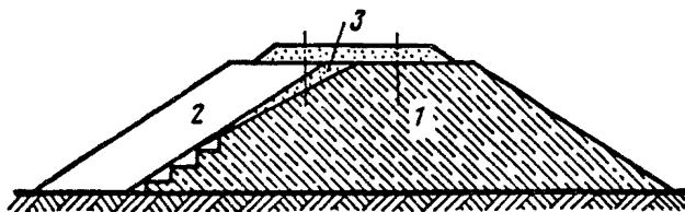
Рис. П.8.53. Деформации насыпи второго пути в результате увлажнения грунта из балластного шлейфа, защемленного при строительстве второго пути:
