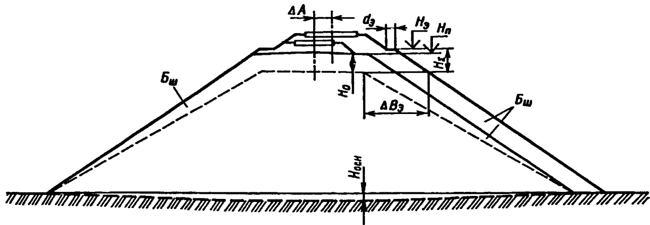
Рис. П.4.2. Высокая насыпь:
