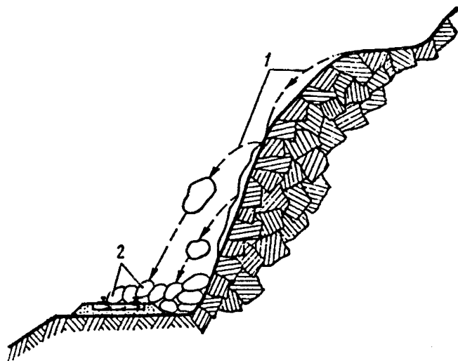
Рис. П.8.19. Обвалы:
