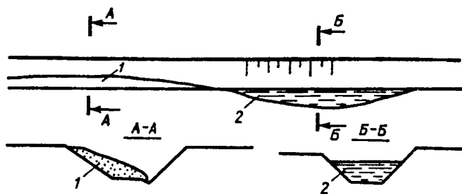
Рис. П.8.41. Понижения и заплывания водоотводов земляного полотна на вечномерзлых грунтах:
