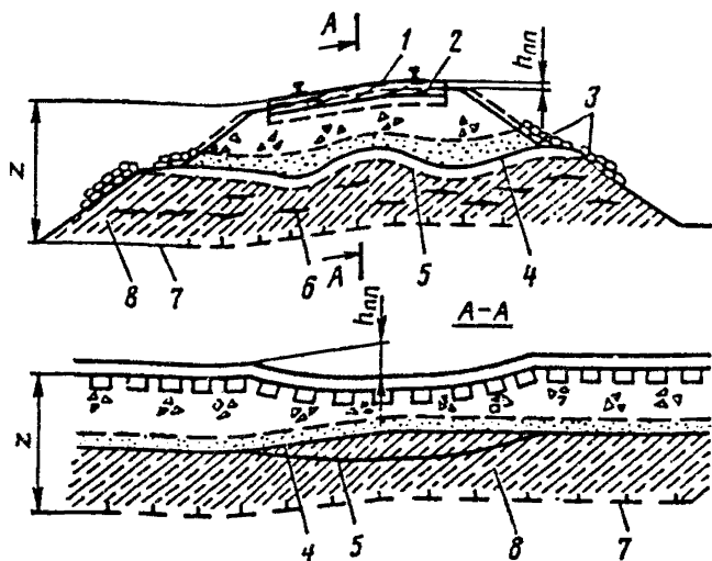
Рис. П.8.6. Весенние пучинные просадки:
