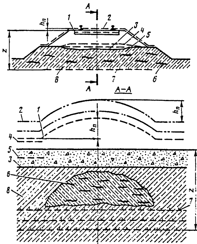
Рис. П.8.7. Пучины:
