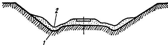
Рис. П.8.57. Уменьшение сечения построечных кюветов: 1 — построечное положение кювета; 2 — положение кювета после подьемки пути
