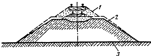
Рис. П.8.21. Оседание насыпи вследствие уплотнения слагающих ее грунтов:
