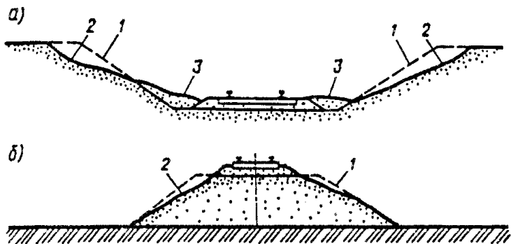
Рис. П.8.38. Развевание песчаных откосов (бровок) в пустынях и полупустынях:
