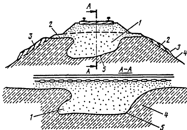
Рис. П.8.3. Балластный мешок:
