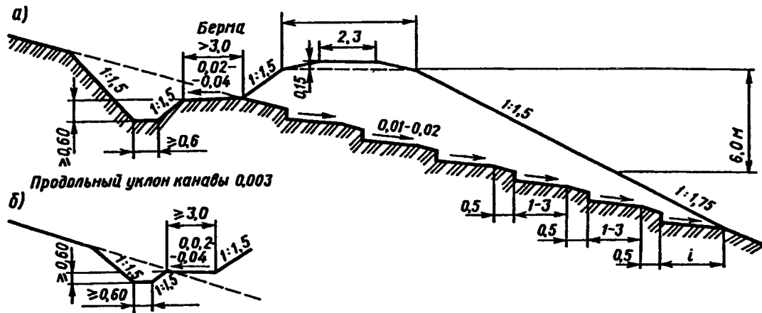
Рис. П.3.5. Насыпи на косогорах
