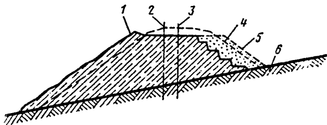
Рис. П.8.23. Сдвиг (сползание) насыпи или ее низовой части по наклонному основанию:
