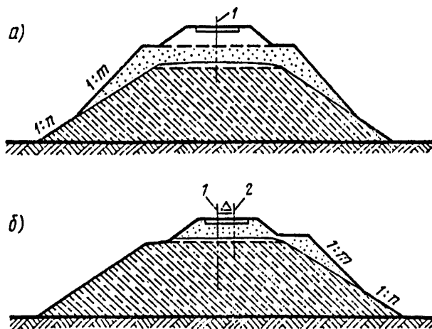
Рис. П.8.55. Балластный шлейф с завышенной крутизной откосов:
