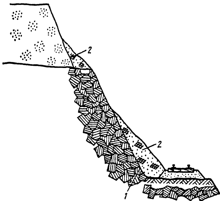
Рис. П.8.17. Осыпи: 1 — откос выемки; 2 — материал осыпи
