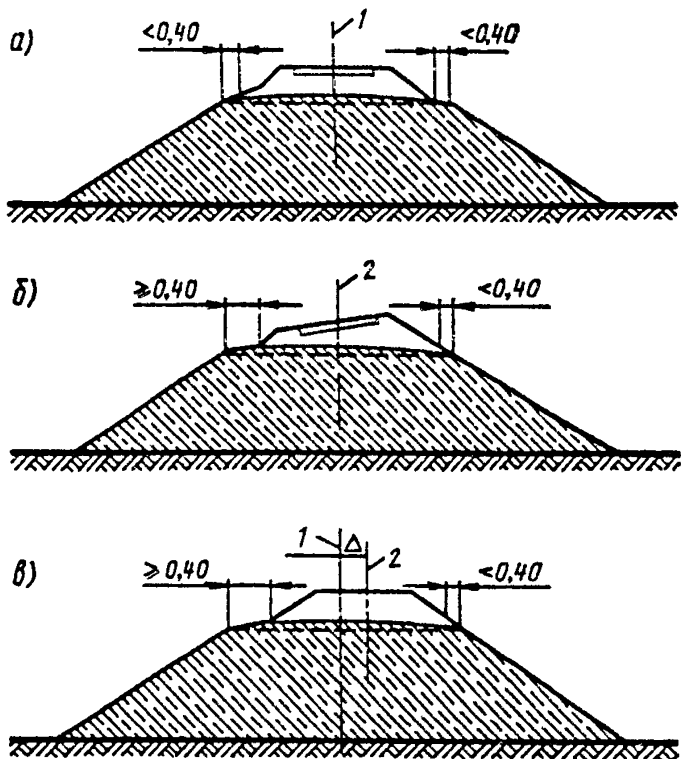
Рис. П.8.54. Недостаточность ширины обочин: a — двусторонняя недостаточность ширины обочин; б — односторонняя недостаточность ширины обочин; в — односторонняя недостаточность ширины обочин при сдвиге оси пути; 1 — положение оси пути существующего пути; 2 — ось пути после сдвиги; \Delta — величина сдвиги пути; 0,40 — ширина обочины, м
