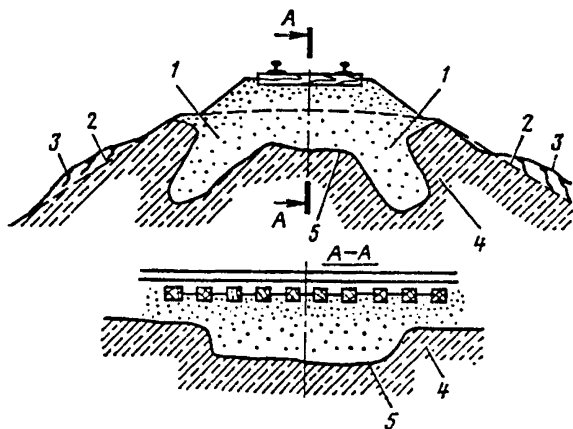
Рис. П.8.4. Балластные гнезда:
