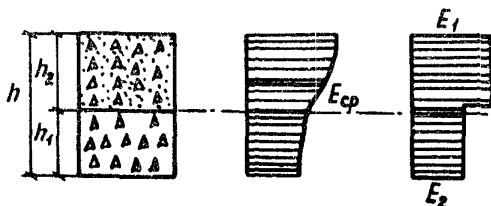
Рис.1. Эюра модулей конструкции щебеночного основания, обработанного в верхней части неорганическими вяжущими: h - общая толщина основания, см; h_1, h_2 - толщины верхней обработанной и нижней необработанной частей слоя основания, см; E_1, E_2 - модули упругости обработанной и необработанной частей слоя основания, МПа; E_{ср} - средний модуль упругости слоя основания, МПа
