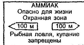
Знак пересечения с несудоходными водными преградами
