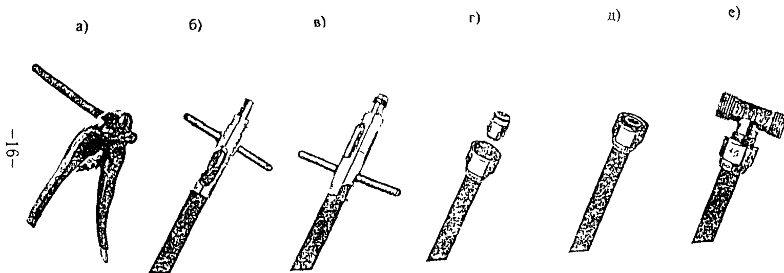
Рис.6.Соединение МПТ с обжимным кольцом и накладной гайкой из латуни:
