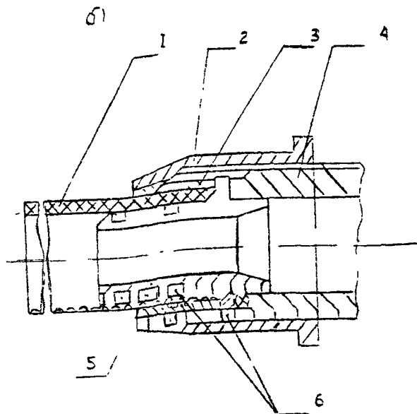
Рис.5.Соединение МПТ с обжимным кольцом и накладной гайкой:
