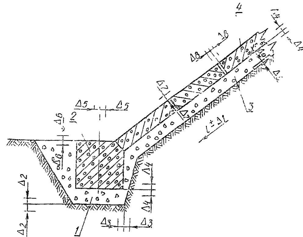
Рис. 2. Схема укрепления откоса насыпи железобетонными плитами:
