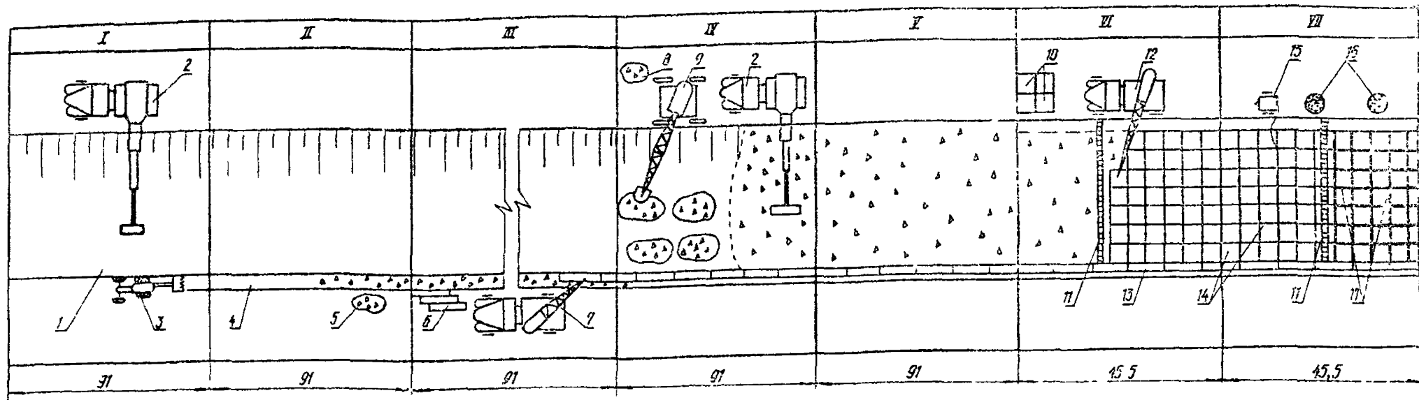
Рис. 1. Технологическая последовательность выполнения комплекса работ по укреплению откоса насыпи железобетонными плитами:
