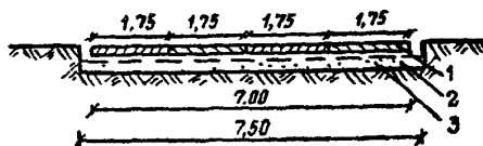
Двухполосное движение
