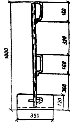
Стойка - ограждение
