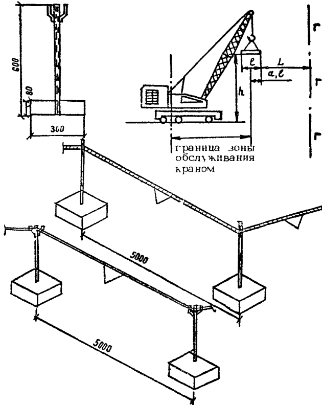
Стойка - ограждение
