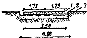
Однополосное движение
