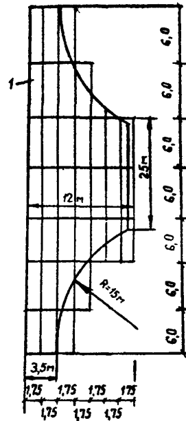
Площадка для стоянки машин
