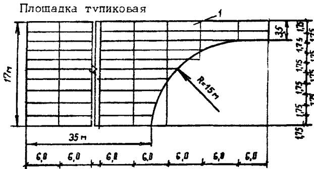
СХЕМЫ ПЛОЩАДОК ДЛЯ СТОЯНКИ И РАЗВОРОТА АВТОМАШИН ПРИ СТРОИТЕЛЬСТВЕ ВРЕМЕННЫХ ДОРОГ
