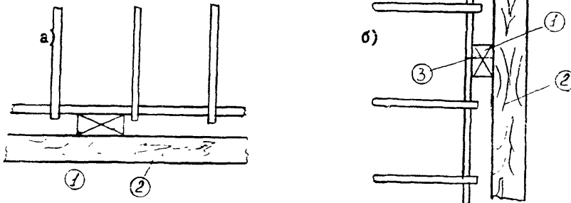
Рис.5 Установка подкладок для обеспечения защитного слоя.
