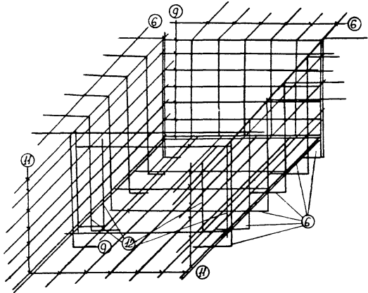
Рис. 3 Наружный каркас прямоуго № 2
