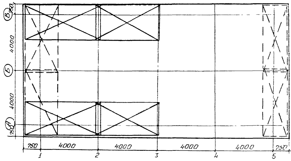
Рис. 6. Схема раскладки сеток C 5
