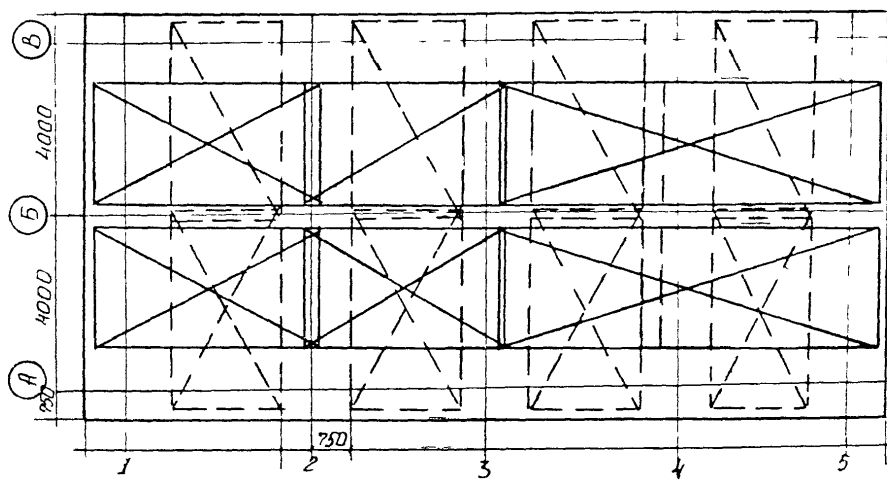
Рис. 8. Схема раскладки сеток С 1 и С 2
