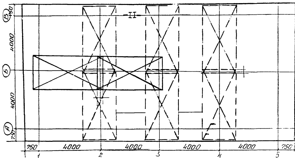
Рис. 6. Схема раскладки сеток C 5
