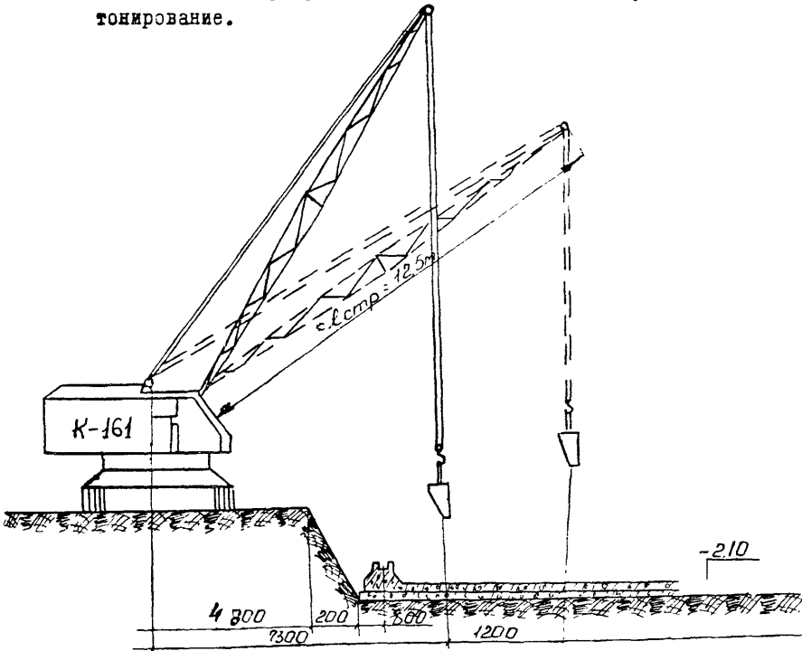
Рис. 10 Подача бетона к рабочему месту
