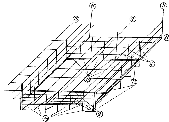
Рис. 2 Внутренний каркас прямка № I
