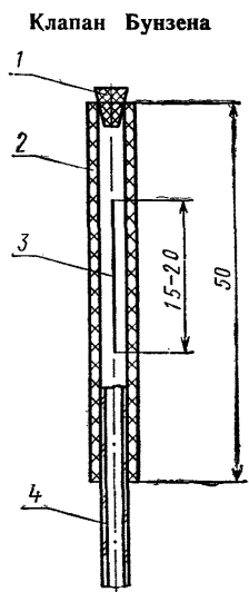
1 — пробка; 2 — резиновая трубка; 3 — щель; 4 — стеклянная трубка Черт. 1
