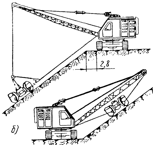
Рис. 1. Планировка откосов двухотвальным планировщиком:
