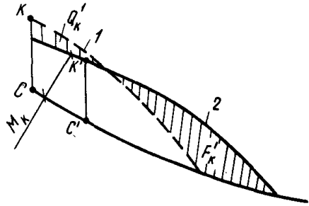
Рис. 14. Схема изменения рельефа в нижней части оползня 1, 2 – рельеф соответственно до и после оползневой подвижки
