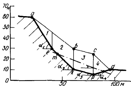
Рис. 25. Схема к расчету устойчивости
