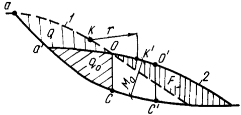
Рис. 15. Схема изменения рельефа в пределах всего тела оползня 1, 2 – рельеф соответственно до и после оползневой подвижки
