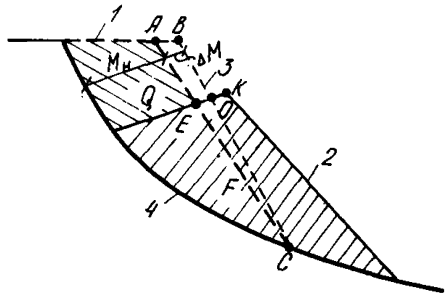
Рис. 16. Схема положения приведенного профиля рельефа 1, 2 – рельеф соответственно до и после оползневой подвижки; 3 – приведенный профиль рельефа
