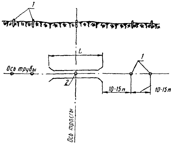
Рис. 1. Схема закрепления местоположения трубы на трассе:
