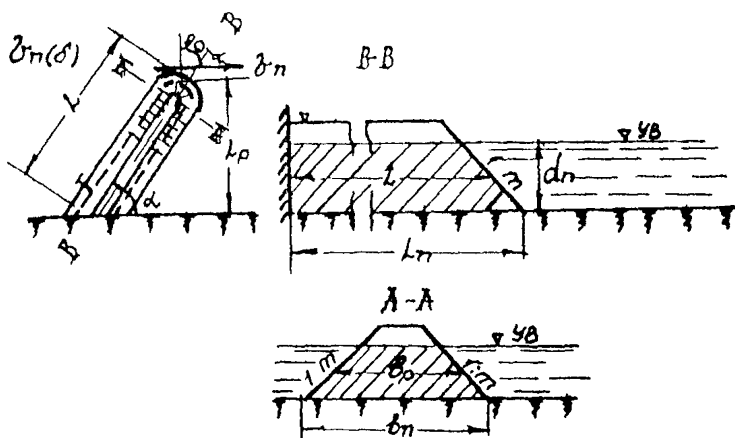
Рис. 10. Траверс у пойменной насыпи
