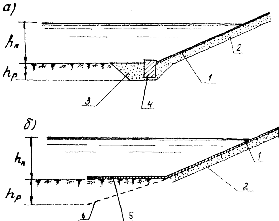
Рис. 7. Защита подошвы откоса:
