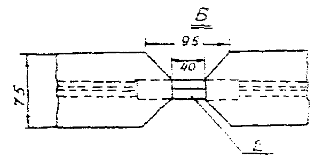
Рис. 5. Гирлянда железобетонного решетчатого покрытия: 1 - петли для стыкования диаметром 12 мм, длиной 464 мм; 2 - полиэтиленовая оболочка толщиной 2 мм, длиной 115 мм; 3 - пазы линейных шарниров
