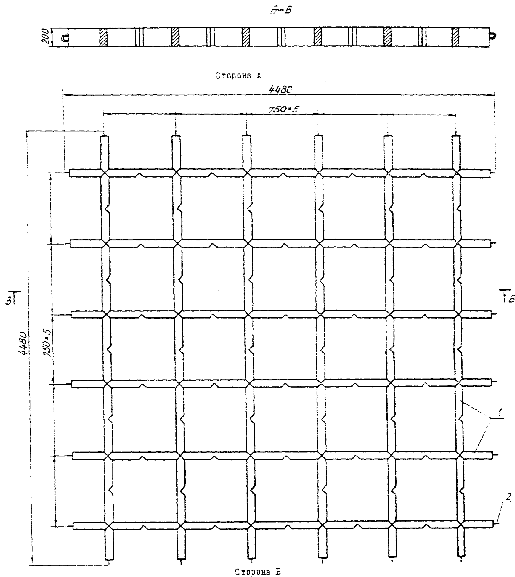
Рис. 4. Блок решетчатого покрытия: 1 - гибкая железобетонная герляда сечением 20,0×7,5 см; 2 - петли для стыкования диаметром 12 мм, длиной 464 мм
