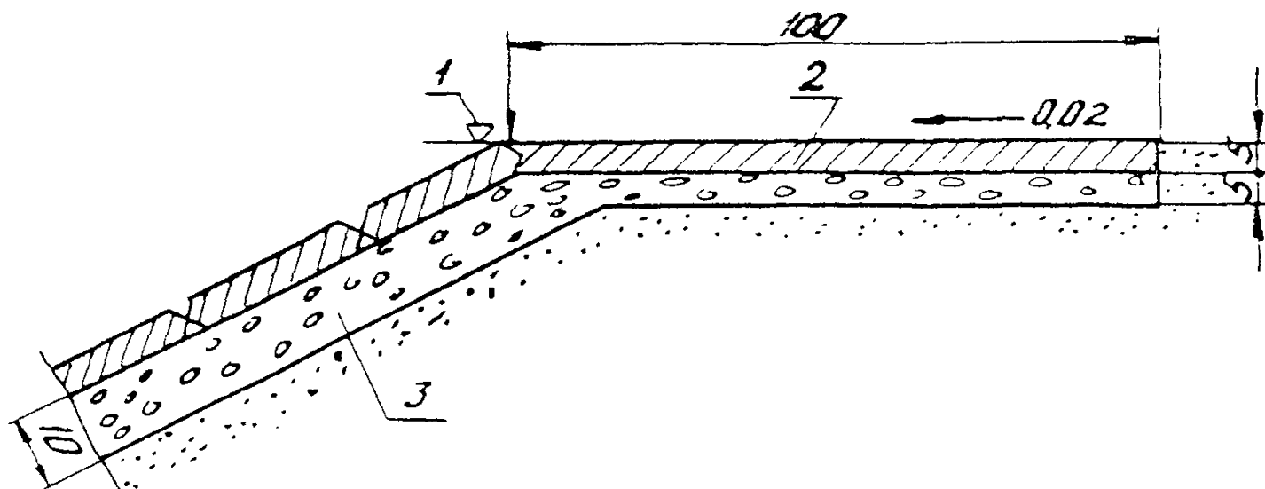
Рис. 8. Сопряжение покрытия с бровкой откоса: 1 - отметка бровки полотна или бермы; 2 - защитный слой; 3 - щебеночно-гравийная подготовка (размеры в сантиметрах)
