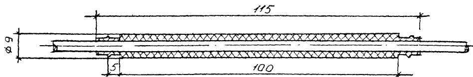
Рис. 1. Полиэтиленовая оболочка стержня арматуры
