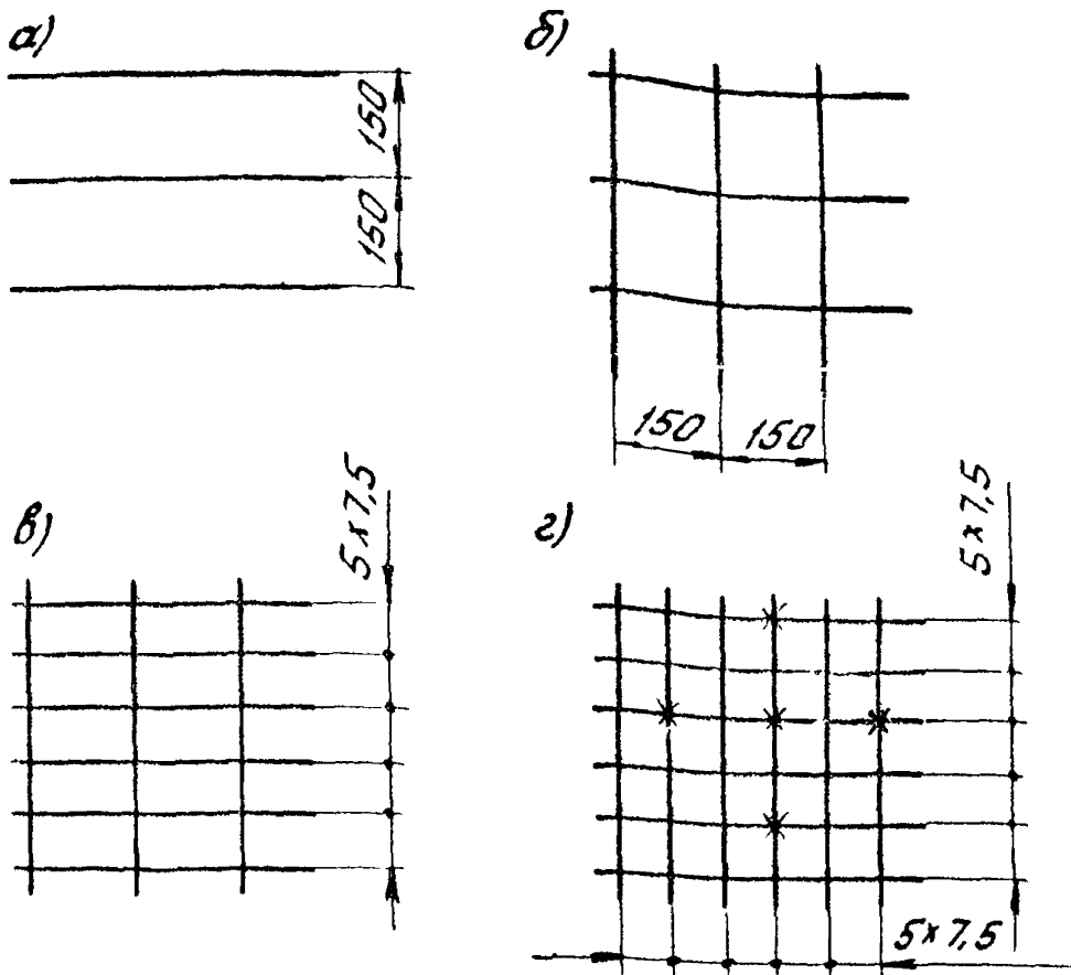
Рис. 13. Приемы раскладки гирлянд в блоке решетки плетением с шагом 75 см:
