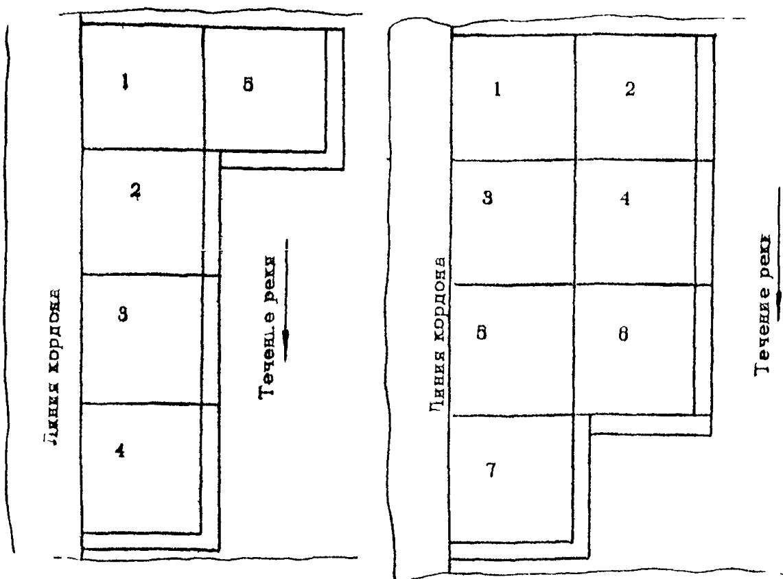
Рис. 14. Последовательность укладки блоков на дно у причала:
