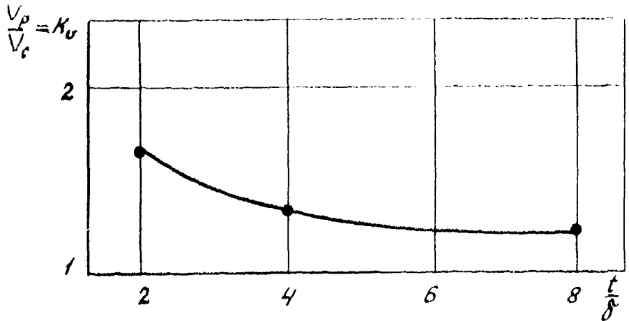
Рис. 9. График определения коэффициента K_v
