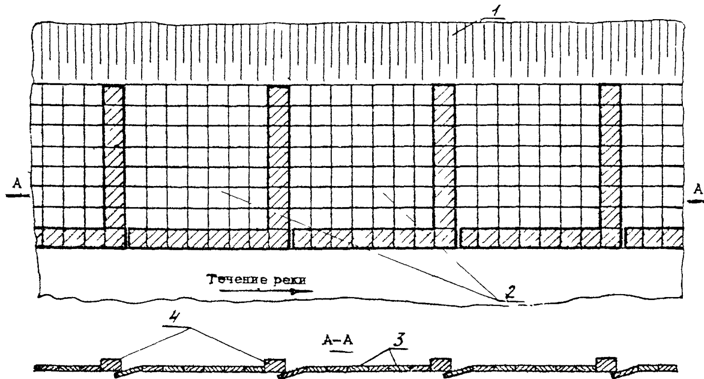
Рис. 3. Схема раскладки плит покрытия: 1 - береговая сторона; 2 - карты покрытия; 3 - железобетонные плиты массой, равной 0,5 расчетной; 4 - железобетонные плиты расчетной массы
