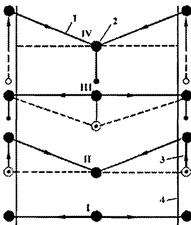
Рисунок 3- Обследование дна водоема по ходовому тросу двумя водолазами
