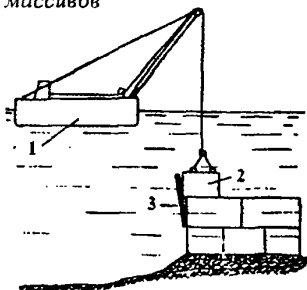
1- плавкран; 2- массив; 3- рейка.
