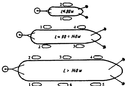
Рисунок 1- Позиция постановки и перемещения водолазного бота при освидетельствовании судна на полизигоне
