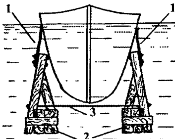
Рисунок 2- Спусковое устройство
