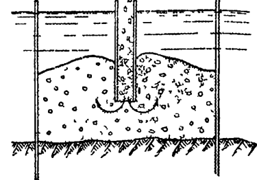
Рисунок 3- Заполнение участка бетоном по способу ВПТ
