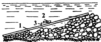
Рисунок 3- Установка реек для наклонной постели
