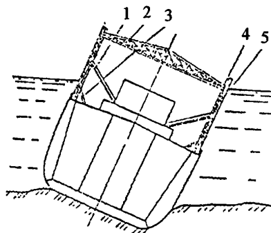
Рисунок 2- Коффердам.
