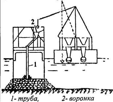
1- труба, 2- воронка Рисунок 2- Схема подачи бетона способом ВПТ
