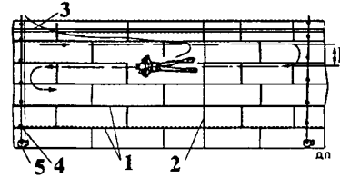
1- пазовые сварные швы; 2- стыковые сварные швы; 3- скуловой киль; 4- маркировочный конец; 5- марка магнитная.
