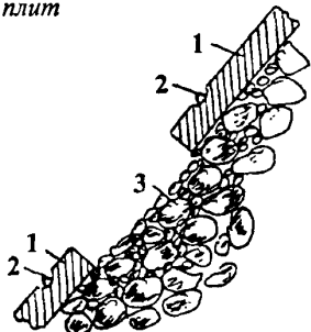
Рисунок 1 - Разборка мощения из плит
