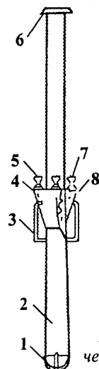
1- крестовина; 2- корпус; 3- ручень; 4- воздушная коробка; 5- гайка заглушка; 6- фланец Ду 150; 7- штуцер подачи воздуха; 8- отверстие для воздуха.
