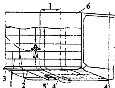
1- пазовые сварные швы; 2- стыковые сварные швы; 3- скуловой киль; 4- подкильный конец; 5- кингстонная решетка; 6- верхняя часть ширстрека.
