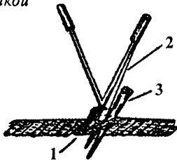
1- перерезаемая прядь троса; 2- ножницы; 3- круглая свайка. Рисунок 4- Резка ножницами стального троса
