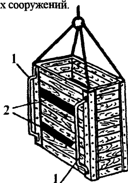
1- опоры; 2- рабочие окна. Рисунок 1- Защитная беседка
