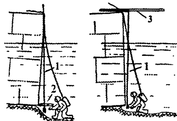
Рисунок 1-Способы обследования гидротехнических сооружений
