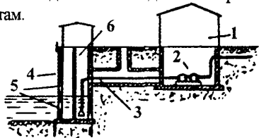
Рисунок 1- Водозаборное сооружение берегового раздельного типа
