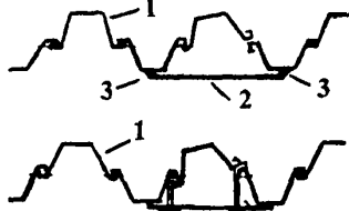
Рисунок 1- Положение зубила при рубке заклепок
