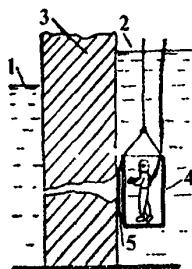
1- нижний бьеф; 2- верхний бьеф; 3- плотина; 4- беседка; 5- опоры. Рисунок 2- Работа водолаза в защитной беседке у стенки
