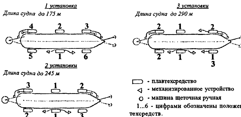
Рисунок 2 - Типовая схема расстановки и перемещения плавсредств с установками при выполнении очистки судна (вариант 2).
