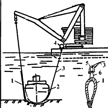
1- подъемный строп; 2- затонувшее судно; 3- проводник; 4- лебедка плавкрана; 5- соединительная скоба; 6- стропка (может отсутствовать).
