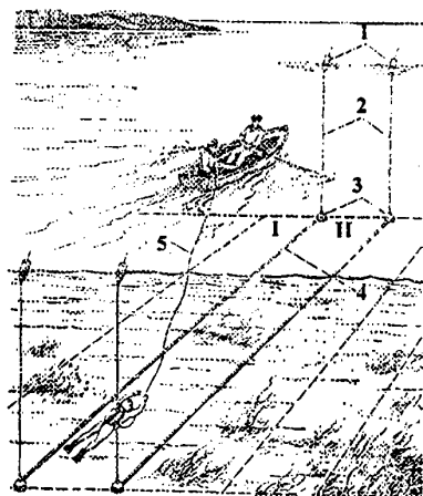
Рисунок 4- Обследование дна полосами
