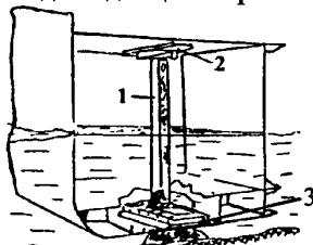
1- распоры; 2- клинья; 3- деревянный щит.
