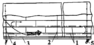
1- пазовые сварные швы; 2- стыковые сварные швы; 3- скуловой киль; 4- маркировочный конец; 5- марка магнитная.
