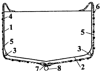
1-борт; 2-днище; 3-скуловой киль; 4-ширстрек; 5-маркировочный подкильный конец; 6- марка; 7- скоба такелажная; 8-груз.
