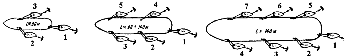
Рисунок 1- Позиции водолазного бота у аварийного судна
