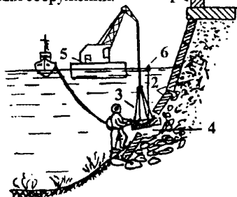
Рисунок 1 - Разборка мощения из плит
