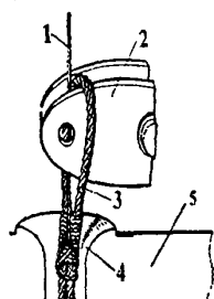
1-шкентель; 2-коромысло; 3- строп; 4-клюз 400-тонного понтона; 5-пonton. Рисунок 2- Застежка стропа 400-тонного понтона на коромысло
