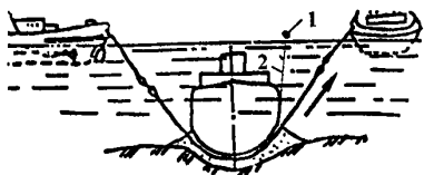
1- буйёк; 2- проводник.
