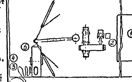
СХЕМА РАССТАНОВКИ ИСПОЛНИТЕЛЕЙ ПРИ ПОСТАНОВКЕ ВЕХИ МЕТОДОМ БУКСИРОВОЙ
