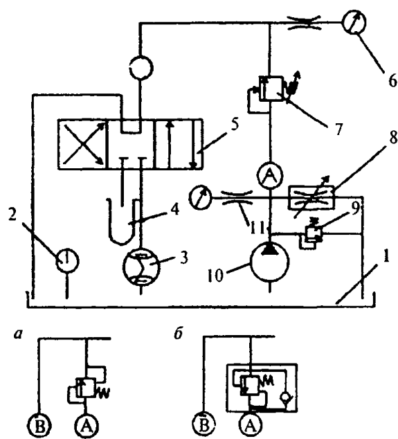
1 — бак, 2 — термометр, 3 — расходомер, 4 — черный сосуд, 5 — распределитель, 6 — манометр, 7 — испытуемый аппарат, 8 — дроссель, 9 — предохранительный клапан, 10 — насос, 11 — кран-демпфер
