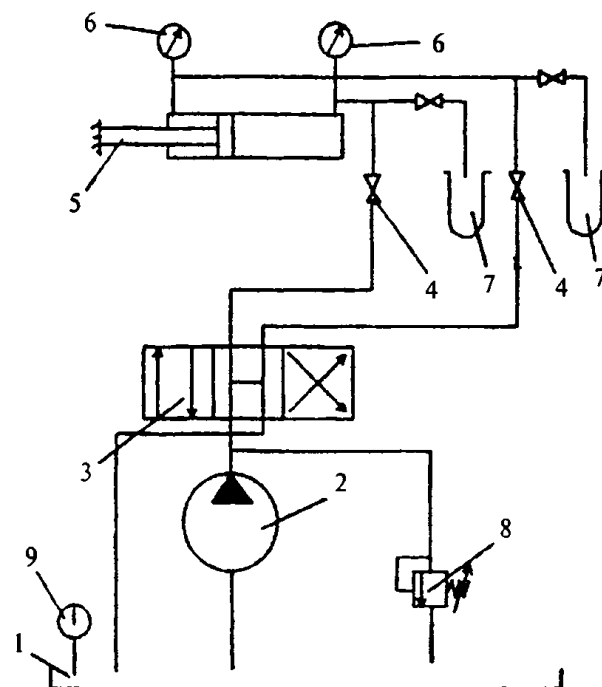
1 — бак, 2 — насос, 3 — распределитель, 4 — вентиль, 5 — испытуемый гидроцилиндр, 6 — манометр, 7 — мерные сосуды, 8 — предохранительный клапан, 9 — термометр
