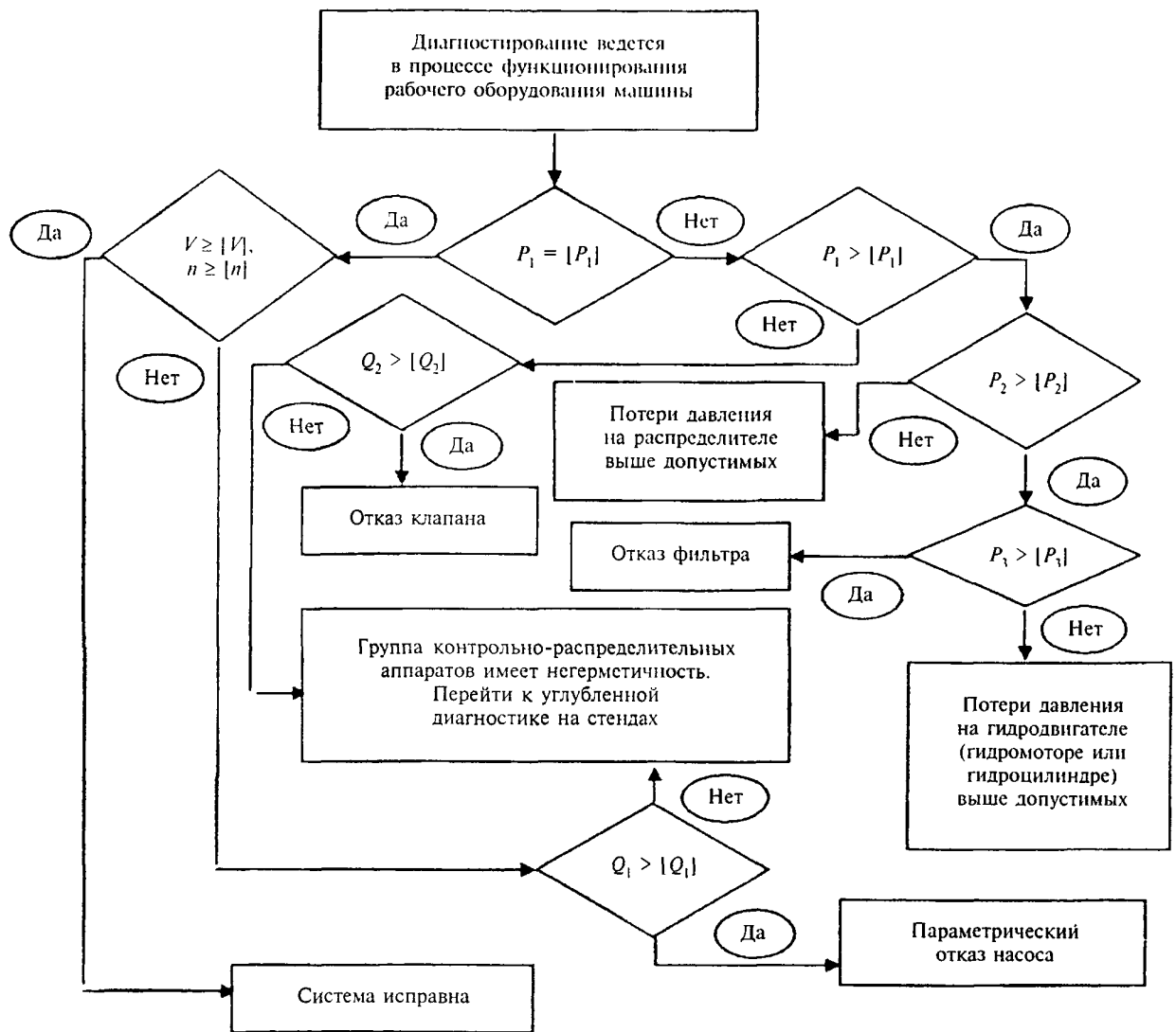
Рисунок 8 – Типовой алгоритм диагностирования гидросистемы в рабочем режиме
