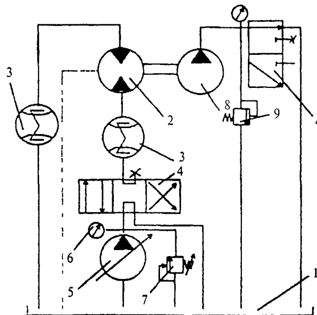
1 — бак, 2 — испытуемый гидромотор, 3 — расходомер, 4 — распределители, 5 — насос, 6 — манометр, 7, 9 — предохранительные клапаны, 8 — нагрузочный насос
