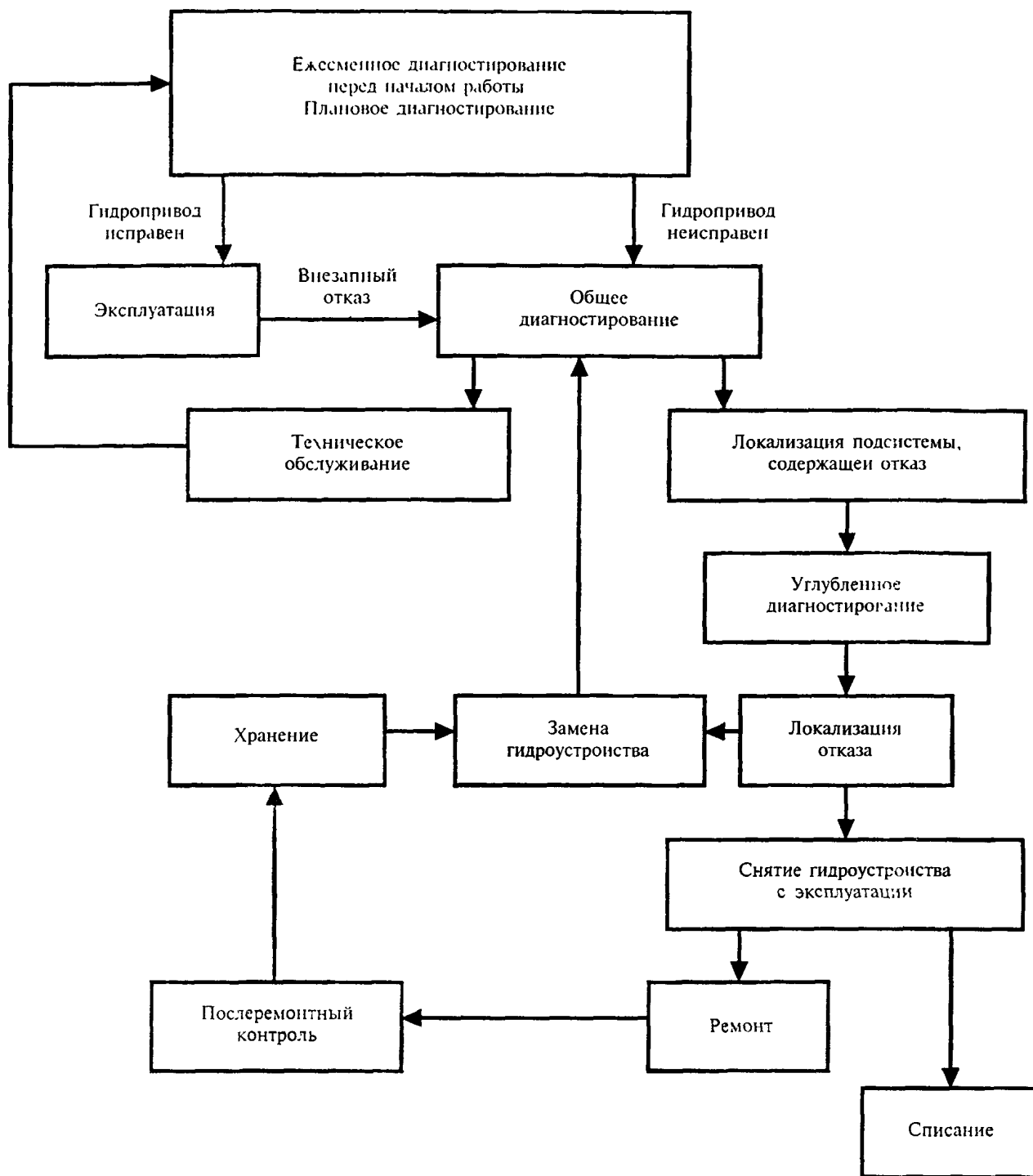
Рисунок 9 — Схема взаимодействия ремонтно-профилактических воздействий на строительную машину при применении диагностирования
